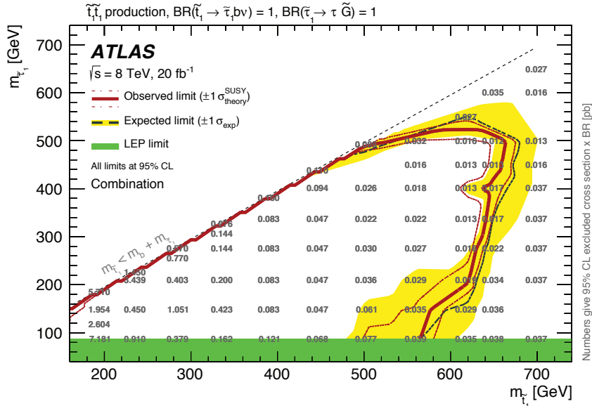
Figure S.3: Uitsluitings limieten voor de top squark productie in het directe verval \tilde{t} \rightarrow \tilde{\tau} b \nu_{\tau} en \tilde{\tau} \rightarrow \tau \tilde{G} bij \sqrt{s} = 8 TeV. De limieten op de \tilde{t} \rightarrow \tilde{\tau} productie werkzame doorsnede worden vermeld in pb voor elke signaal hypothese.
