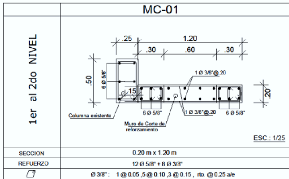
Figura N° 37. Detalle de muros de corte MC-01 (Módulo de Laboratorio y Aulas)
