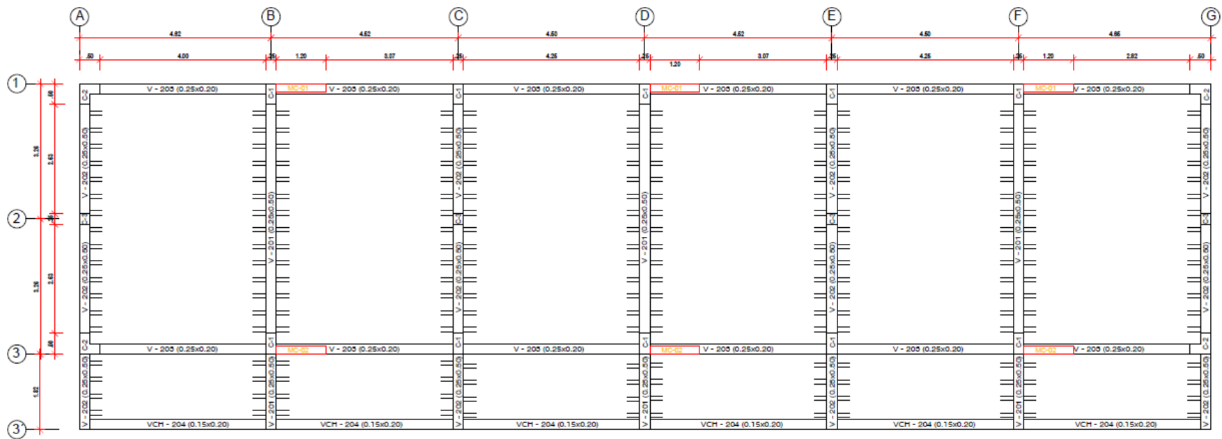
Figura N° 35. Ubicación de muros de corte proyectados para rigidizar la estructura (Módulo de laboratorio y Aulas, segundo nivel) (Eje A-G)
