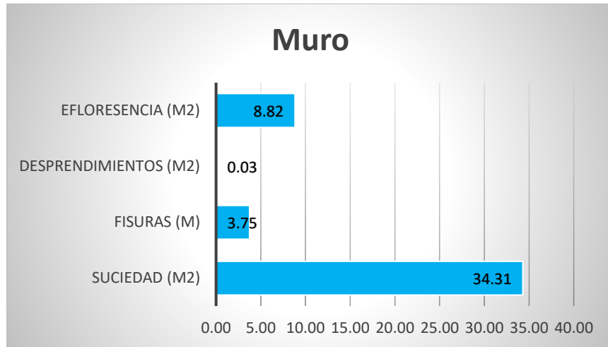
Figura N° 17. Evaluación en vigas Muros del Módulo de Laboratorio y Aulas.
