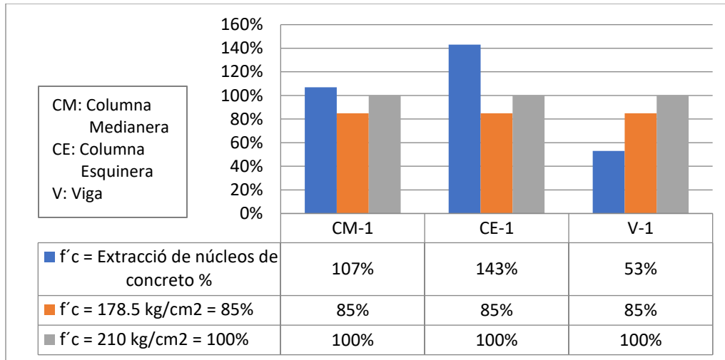
Figura N° 27. Resistencia a la compresión promedio, obteniendo en la rotura de los corazones diamantinos (Módulo de laboratorio y Aulas, primer nivel)
