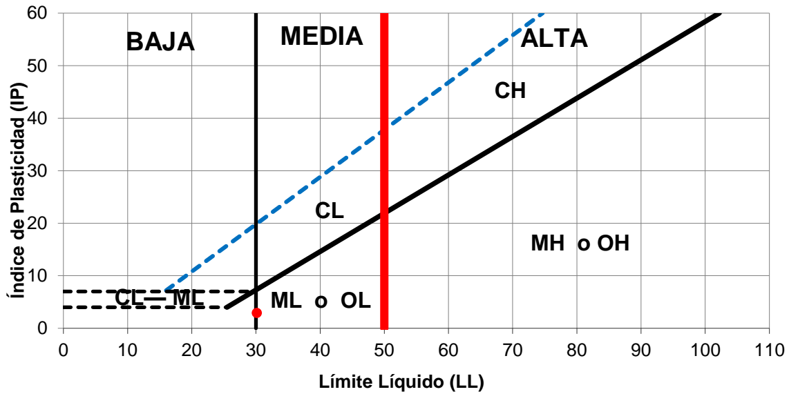
Figura N° 19. Carta de Plasticidad del estrato C -1 de M- 1
