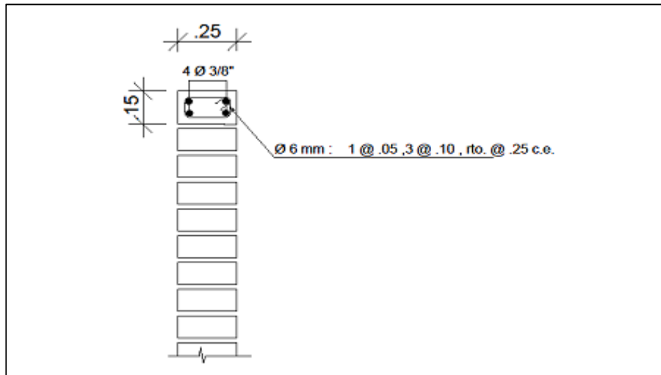
Figura N° 42. Detalle de viga de confinamiento (Módulo de Laboratorio y Aulas)
