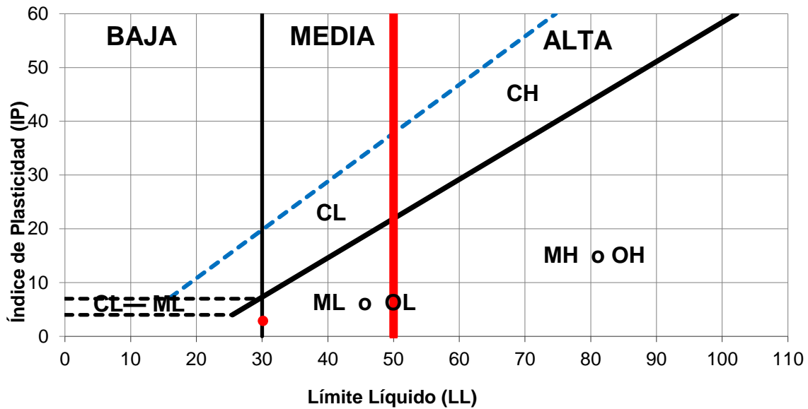
Figura N° 22. Carta de Plasticidad del estrato C -2 de M- 2
