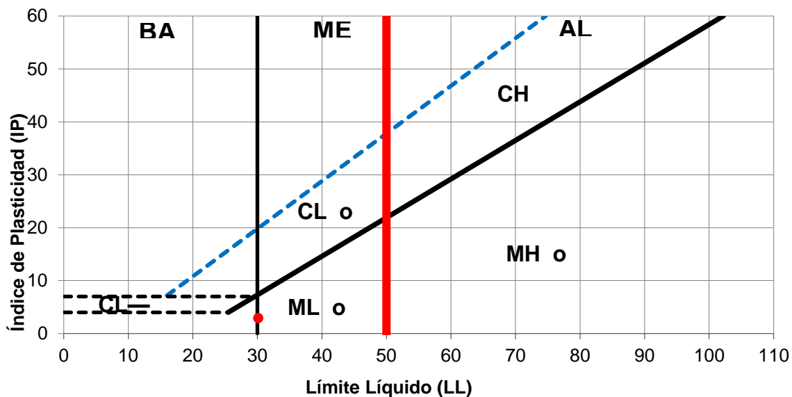
Figura N° 25. Carta de Plasticidad del estrato C -4 de M- 1
