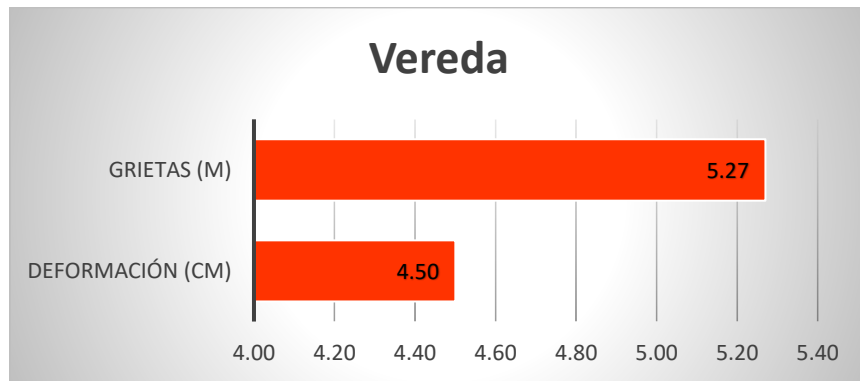
Figura N° 18. Evaluación en veredas Muros del Módulo de Laboratorio y Aulas.
