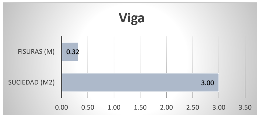
Figura N° 16. Evaluación en vigas del Módulo de Laboratorio y Aulas.
