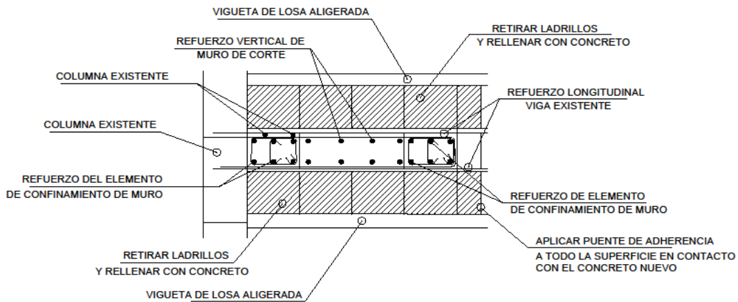
Figura N° 39. Anclaje típico de refuerzo proyectado Viga – Losa – Placa en concreto existente.
