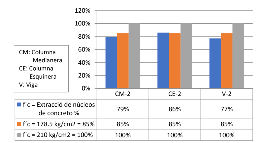
Figura N° 28. Resistencia a la compresión promedio, obteniendo en la rotura de los corazones diamantinos (Módulo de biblioteca y Aulas, primer nivel)
