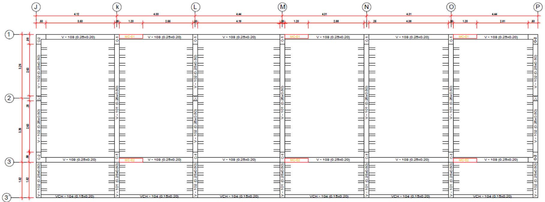
Figura N° 34. Ubicación de muros de corte proyectados para rigidizar la estructura (Módulo de laboratorio y Aulas, primer nivel) (Eje J-P)
