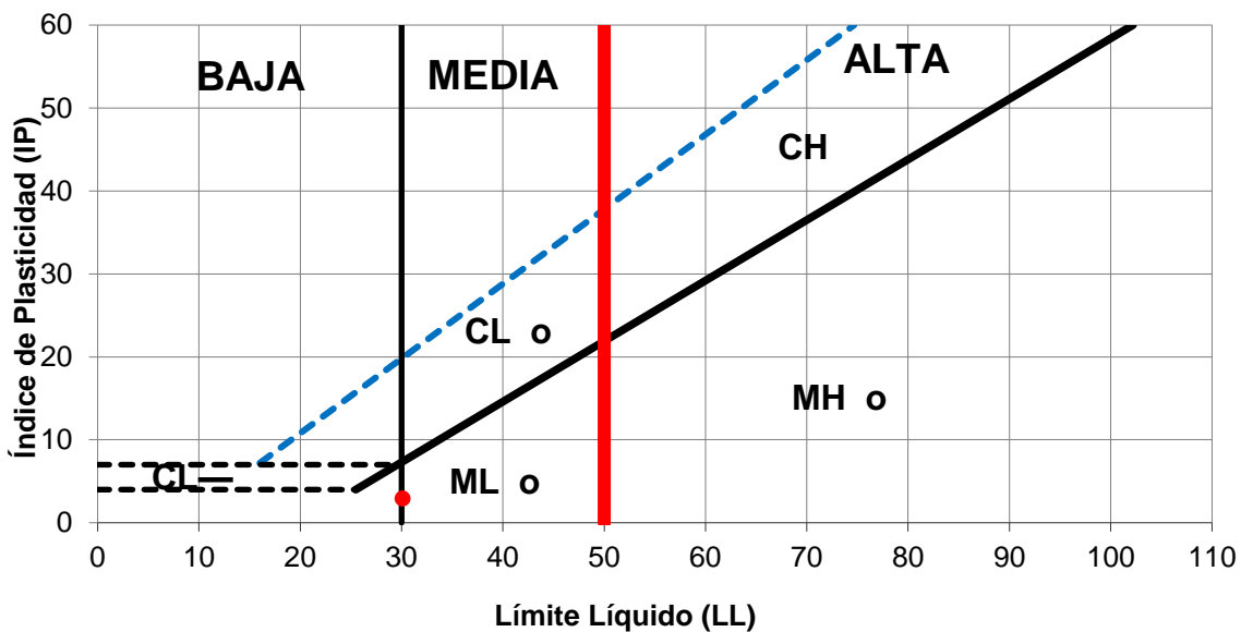
Figura N° 23. Carta de Plasticidad del estrato C -3 de M- 1
