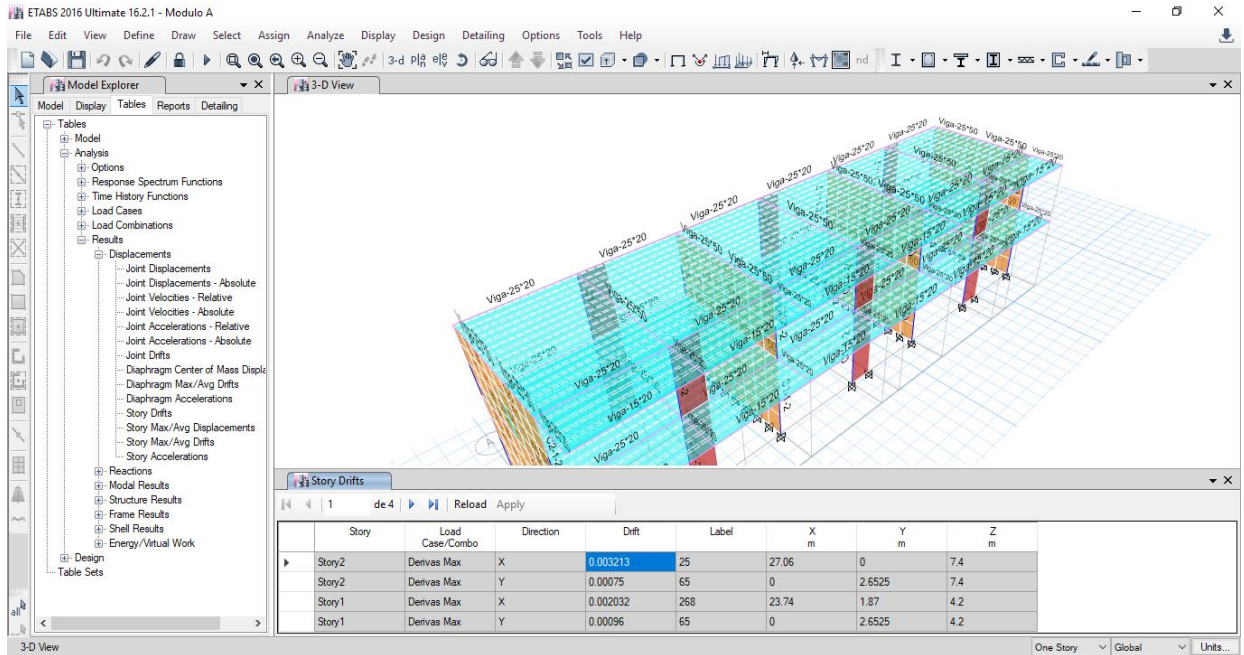
Figura N° 31. Modelamiento de Módulo 1 con Muros de Corte (Diseño con Reforzamiento)
