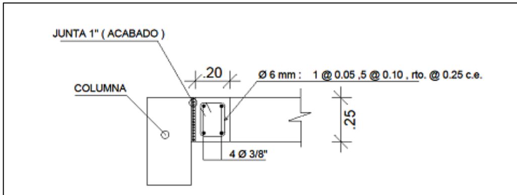
Figura N° 41. Detalle de columna de confinamiento (Módulo de Laboratorio y Aulas)
