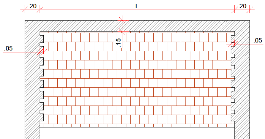
Figura N° 40. Detalle típico de demolición parcial de tabiques (Módulo de Laboratorio y Aulas).
