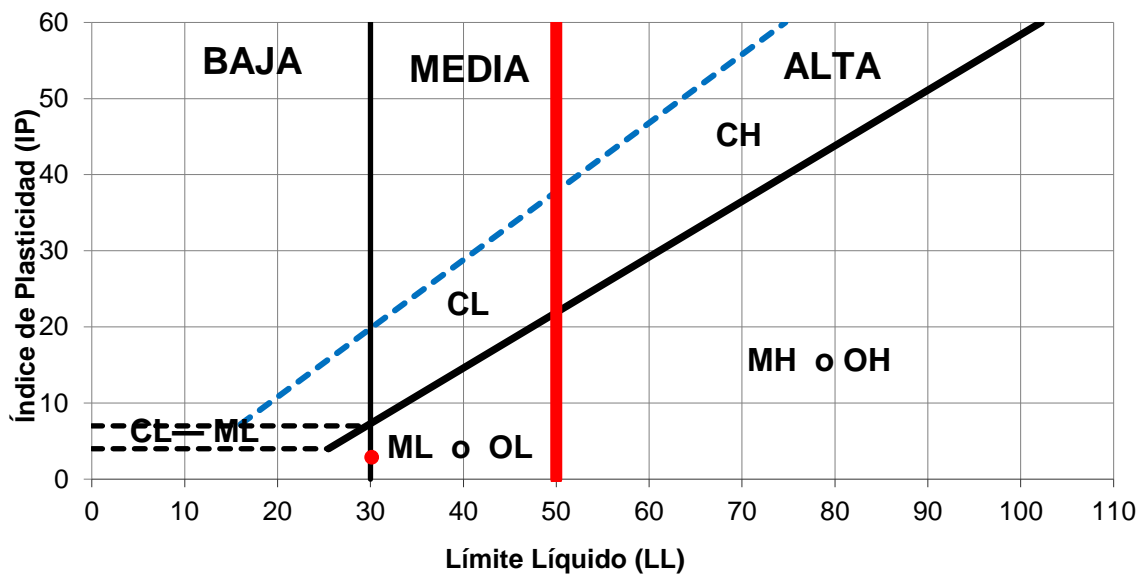
Figura N° 24. Carta de Plasticidad del estrato C -3 de M- 2
