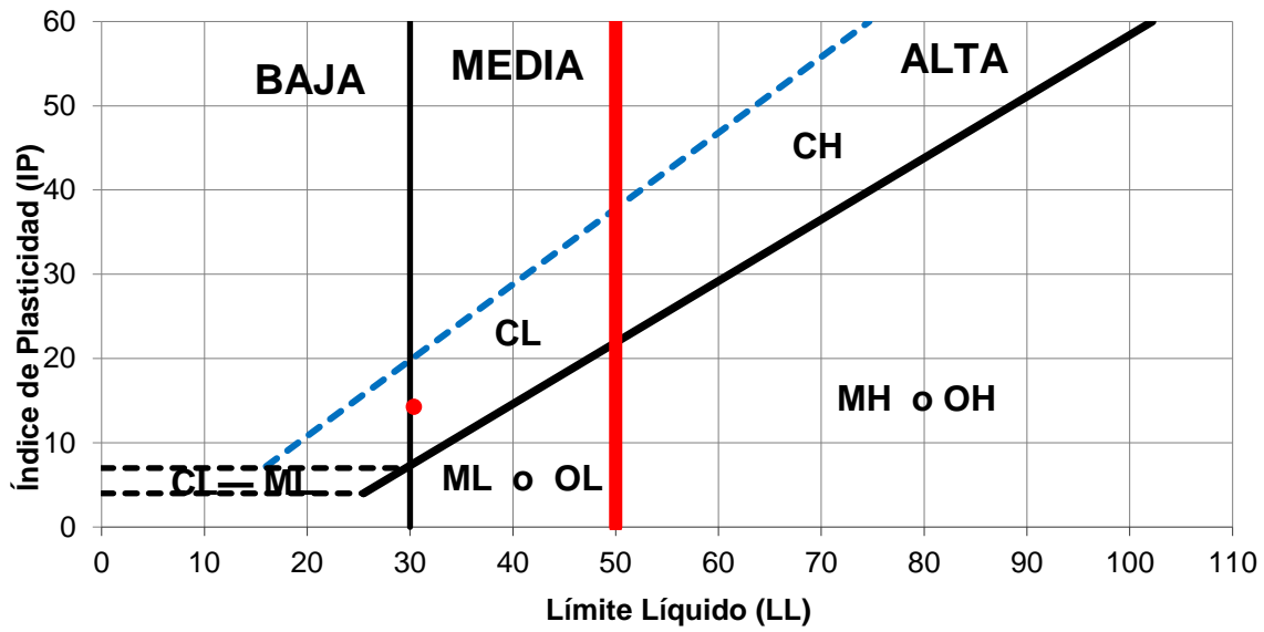
Figura N° 20. Carta de Plasticidad del estrato C -1 de M- 2
