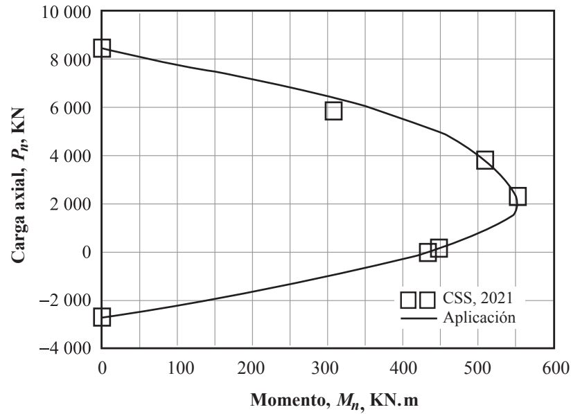
GRÁFICA 5 Curva de interacción nominal en la columna C2 Fuente: Structure Point (2020).
