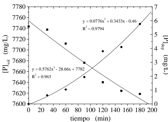
Figura 4 c). Comportamiento del P en disolución del baño de niquelado químico y en el depósito.
