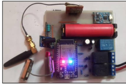
Gambar 10. Hardware wiring pada PCB
