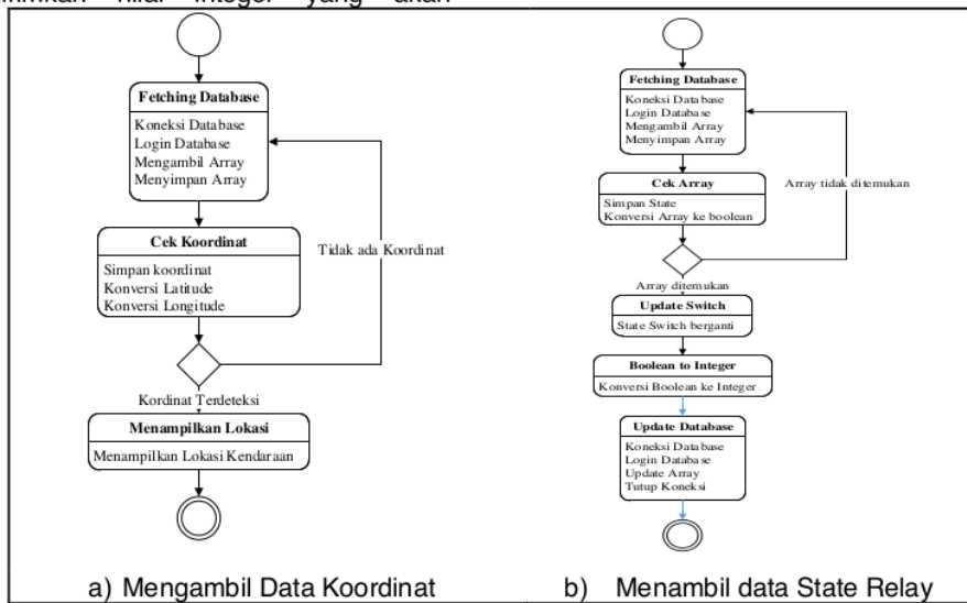
Gambar 7. Statechart Fetch data Koordinat dan State Relay
