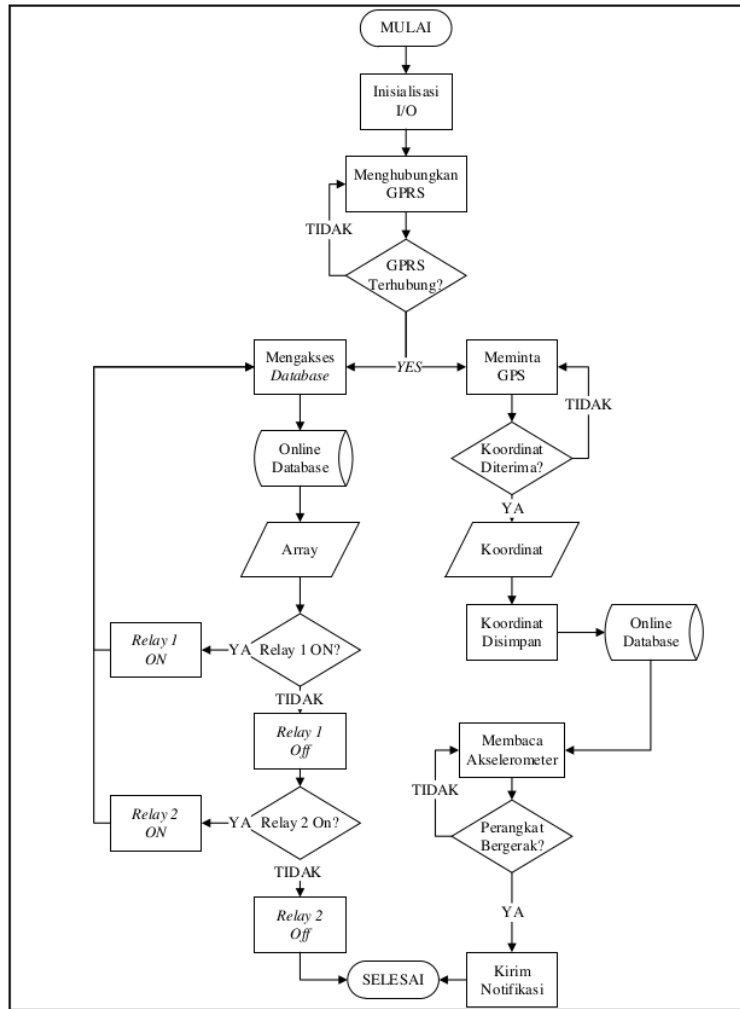
Gambar 4. Flowchart Program Pada Mikrokontroler
