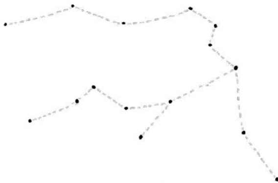
AQUARIUS
