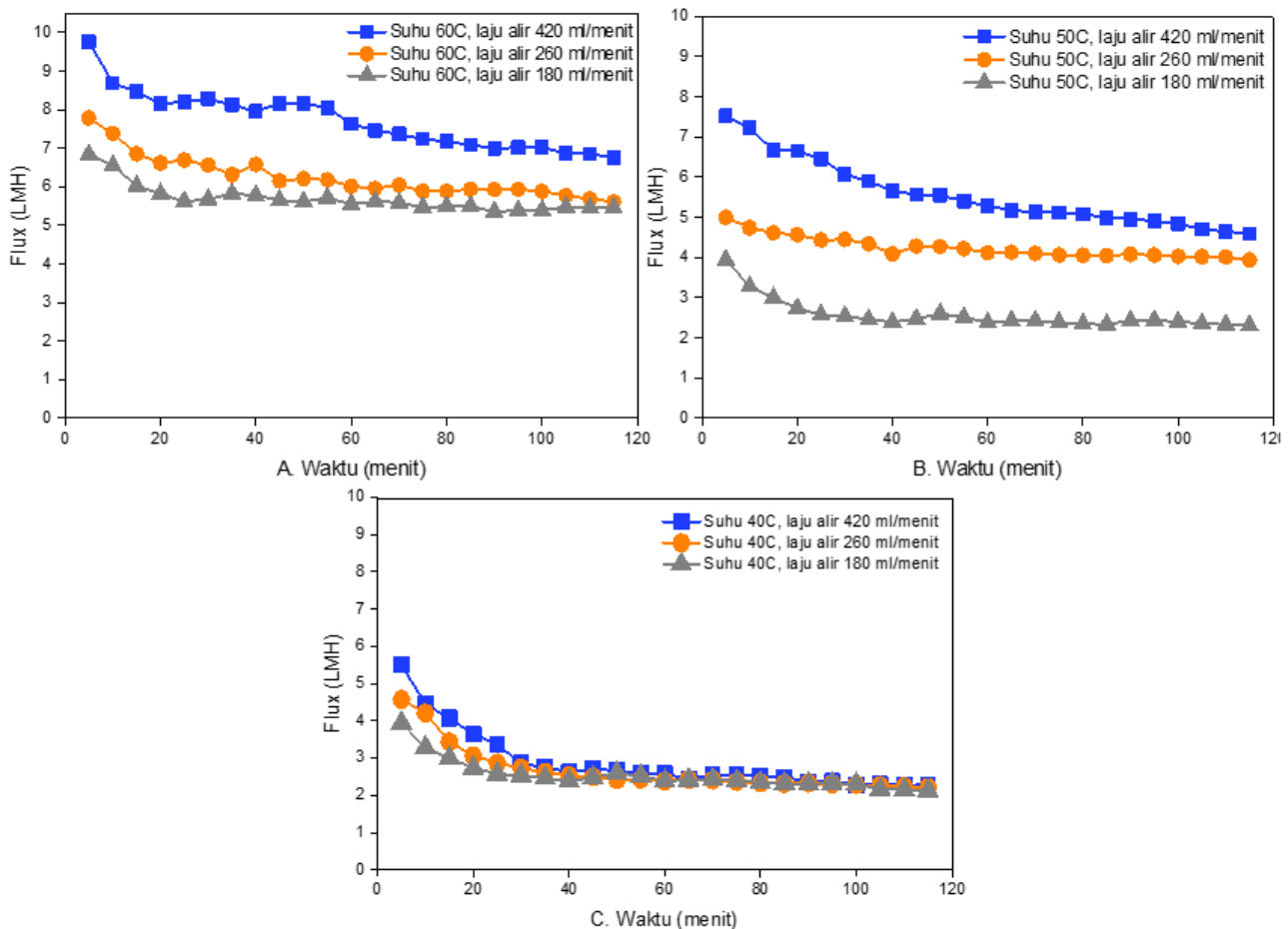
GAMBAR 8. Fluks air dengan variasi laju alir diberbagai suhu operasi.
