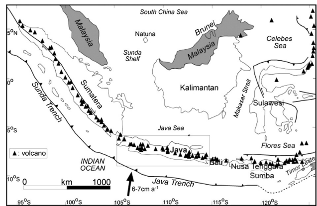
GAMBAR 1. Peta persebaran tektonik dan vulkanik di Indonesia (Purnomo dan Pichler 2014).
