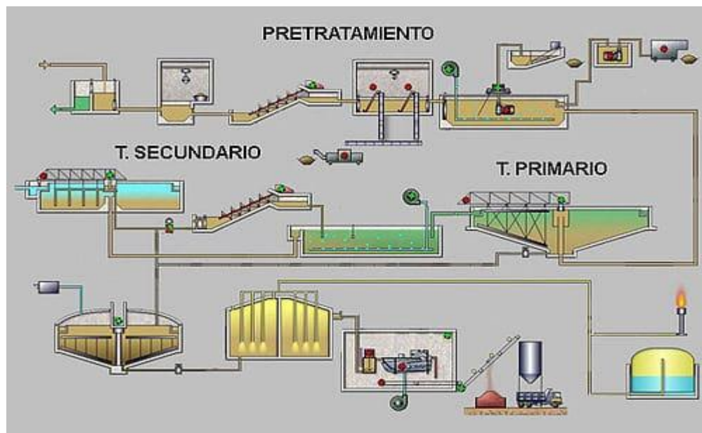
Figura 2. Etapas del proceso de tratamiento
