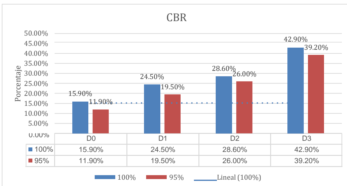
Figura 25. CBR del suelo natural con adición de ceniza de carbón.
