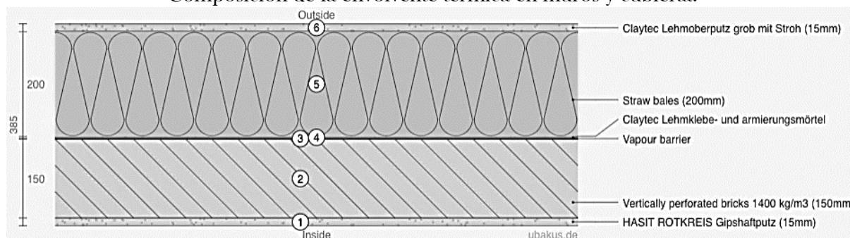
Figura 2. Composición de la envolvente térmica en muros y cubierta.
