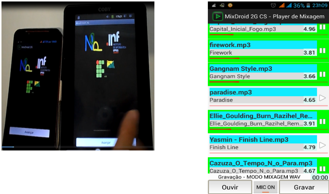
Fig. 1. Metáfora da listra: destaque para a incorporação do processamento de áudio mantendo a simplicidade do mecanismo de interação da marcação temporal.
