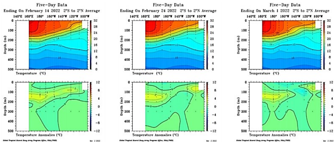
Imagen 3. Corte profundidad vs. Longitud de la temperatura del agua del mar y su anomalía en el Pacífico ecuatorial
