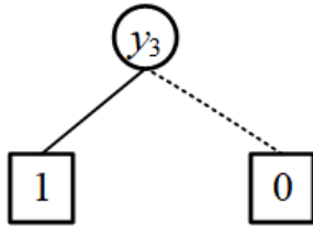
Рис. 4. ROBDD-граф функции f(x_1, x_2, x_3, x_4, 0, 1, y_3)
