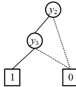
Рис. 5. ROBDD-граф функции f(x_1, x_2, x_3, x_4, 0, y_2, y_3)
