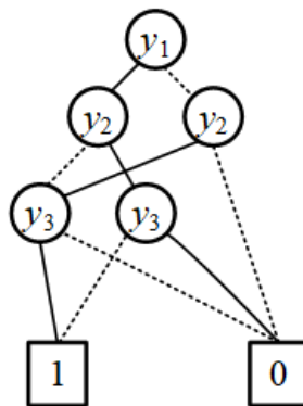
Рис. 6. ROBDD-граф, представляющий все достижимые реакции
