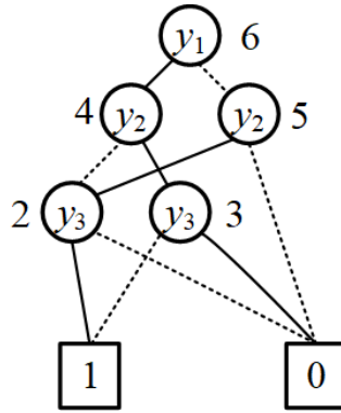
Рис. 3. ROBDD-граф достижимых реакций схемы Fig. 3. ROBDD of reachable circuit patterns
