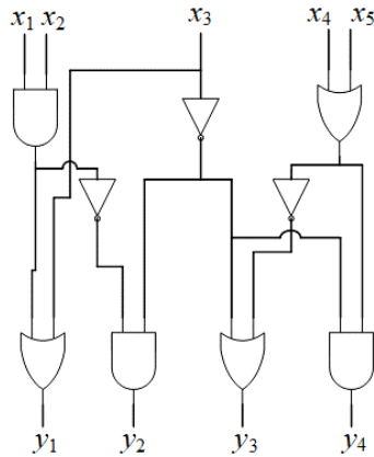
Рис. 1. Пример комбинационной схемы Fig. 1. Example of combinational circuit
