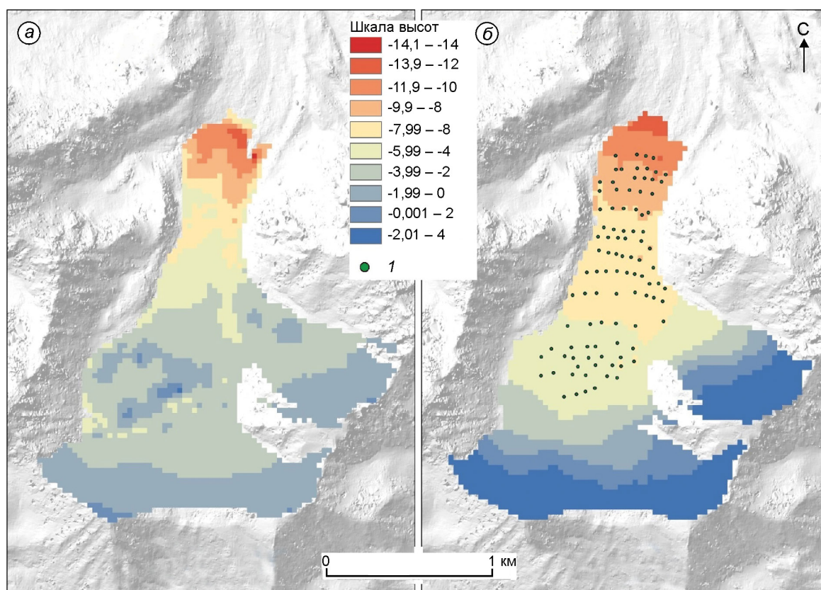
Рис. 5. Результаты изменения баланса массы ледника Центральный Туйыксу (в м.в.э.) за период 2016–2021 гг. полученных геодезическим (а) и гляциологическим (б) методами; I – точки (забуренные рейки).
