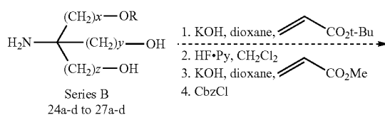
Scheme 29.
