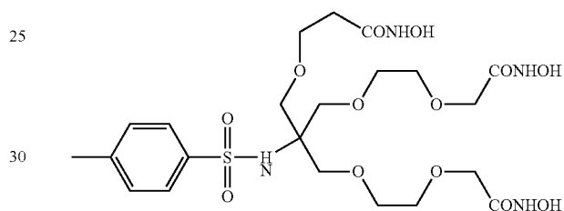
Ligand 6
