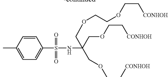
Ligand 5
