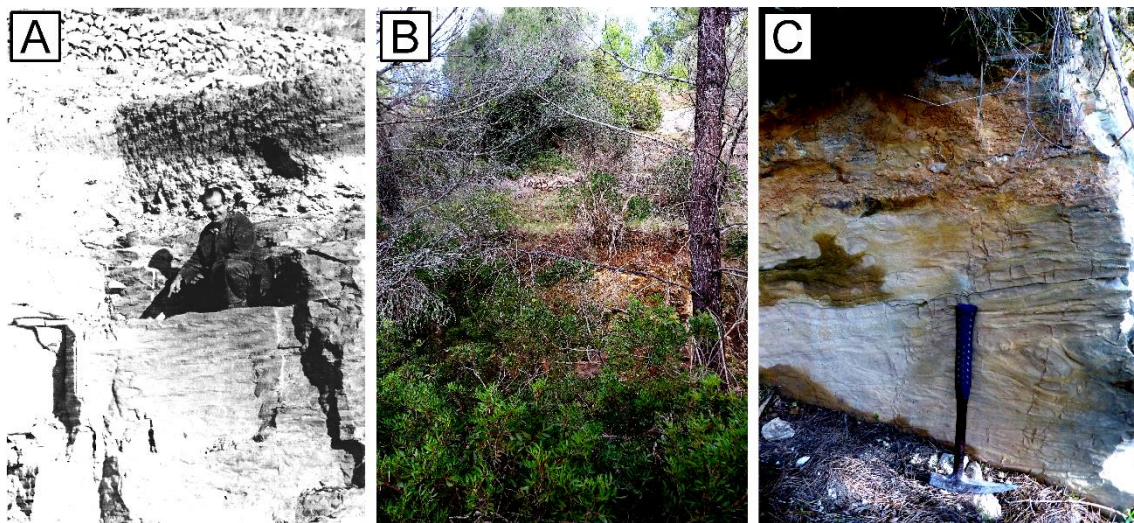
Figura 2. Jaciment de la pedrera de son Dameto (Esporles, Mallorca). A: Fotografia on hi apareix Joan Bauzá assenyalant el suposat nivell de procedència del peix. B: Fotografia actual de la pedrera de son Dameto, corresponent aproximadament a la localització que es mostra a la subfigura A. C: Fotografia actual on es veuen les estructures sedimentàries de la unitat de calcarenites grises dins les que suposadament es va trobar el peix.
