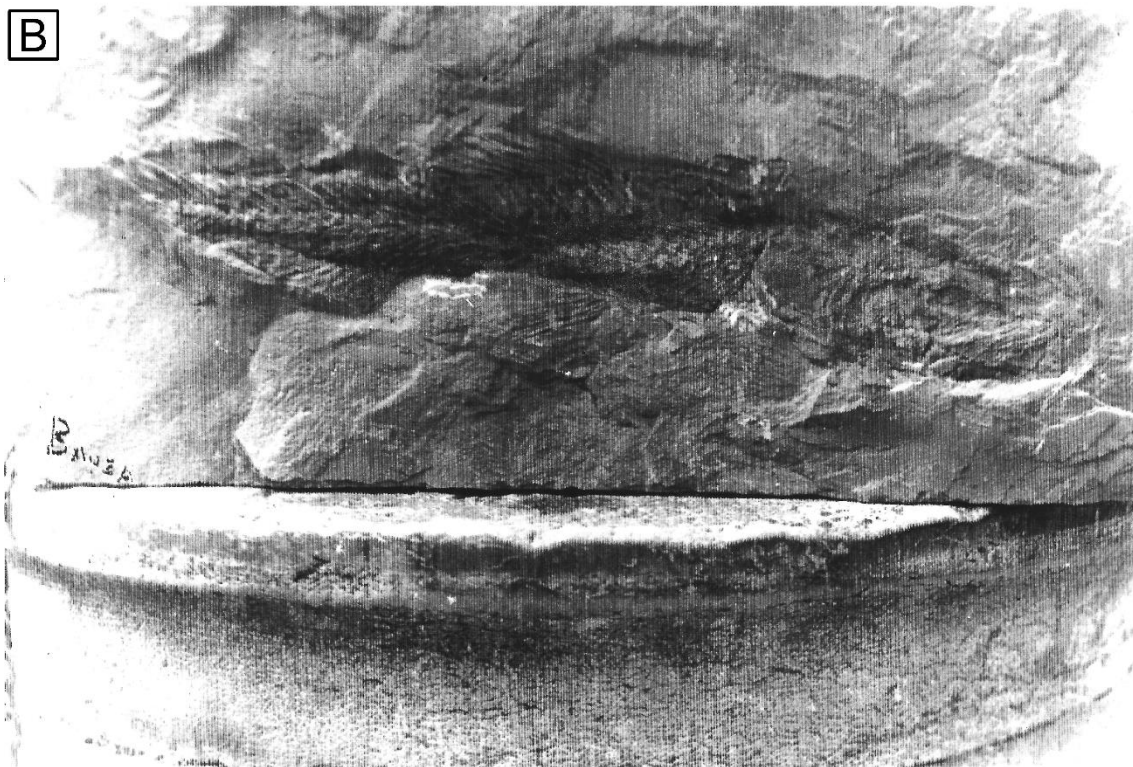
Figura 3A–B. Dues fotografies del teleosti fòssil del Miocè inferior de la pedrera de son Dameto (Esporles, Mallorca).
