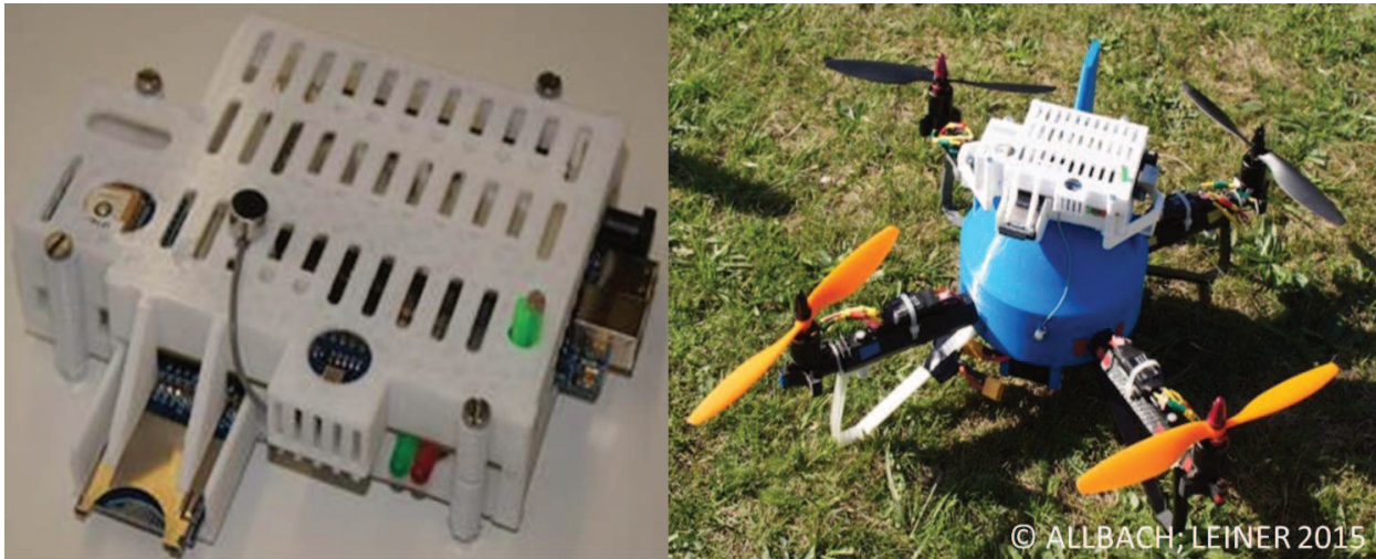
Abb. 2: Mikrocontrollerbasierte Wetterstation & Copter als Trägersystem der Wetterstation [EIGENE DARSTELLUNG, 2014, 2015].
