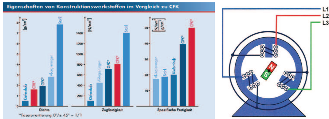
Abb. 1: Werkstoffe & Motor [Quelle: WWW.BENTELER-SGL.DE & BÜCHI, 2013b:16].
