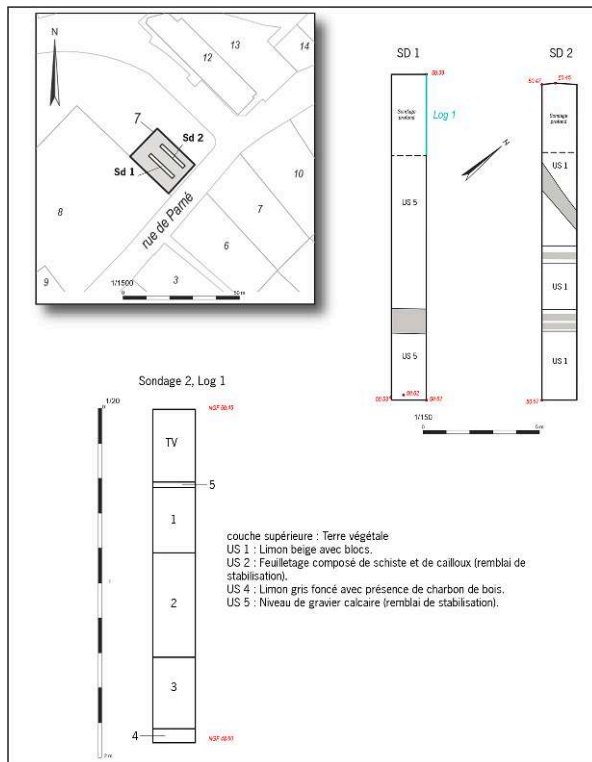
Fig. 1 – Plan général de l'opération
