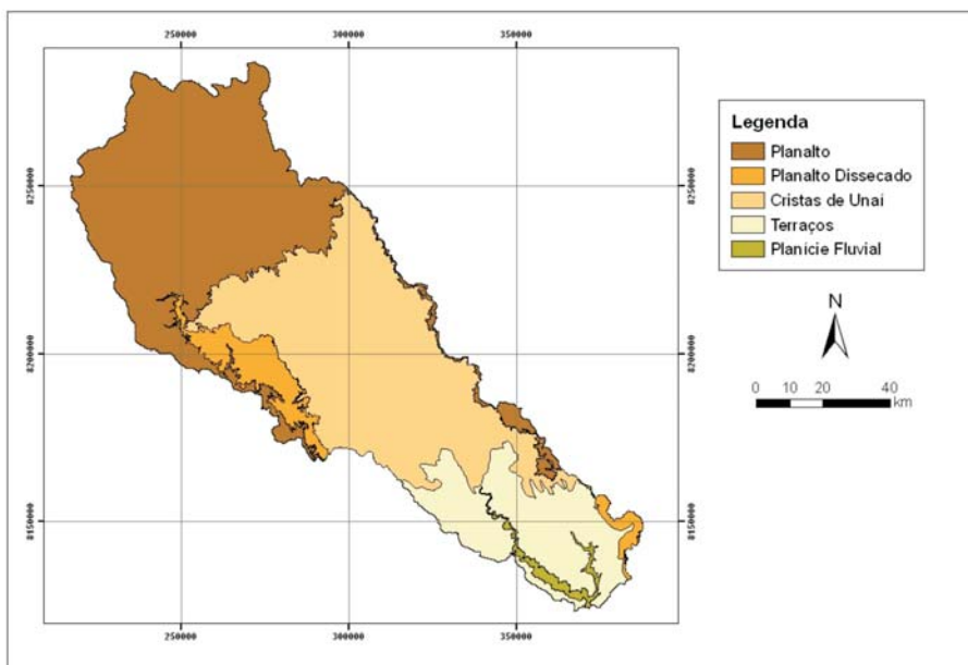
Figura 7 - Compartimentação geomorfológica em primeiro nível da bacia do rio Preto.
