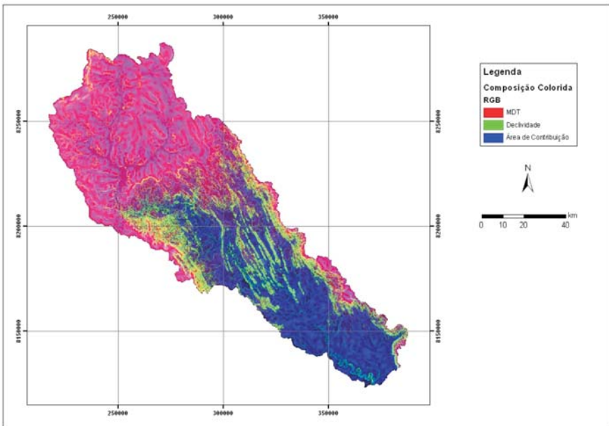
Figura 4 - Composição colorida (RGB): MDT, declividade e área de contribuição.
