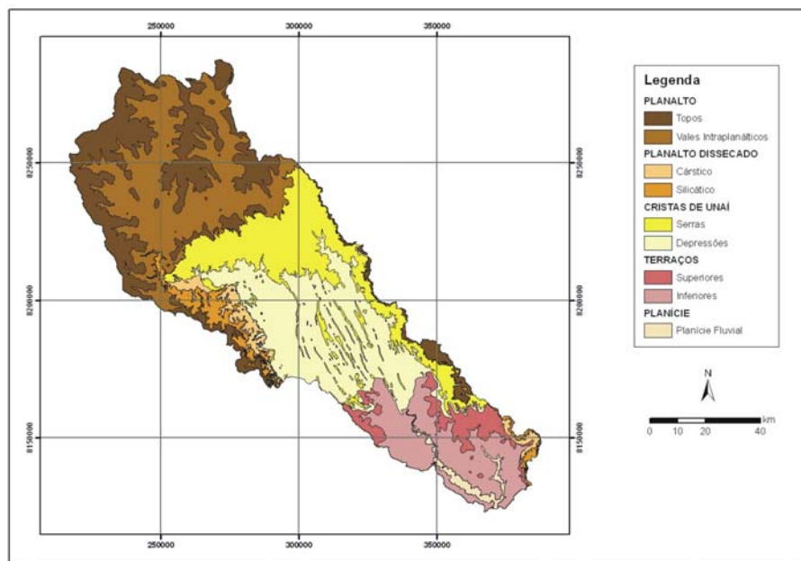
Figura 8. Compartimentação geomorfológica em segundo nível da bacia do rio Preto.
