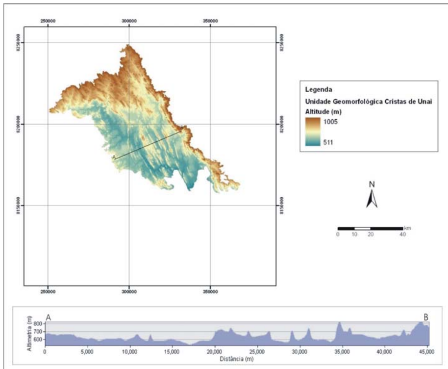
Figura 11 - MDT da unidade geomorfológica Cristas de Unai.
