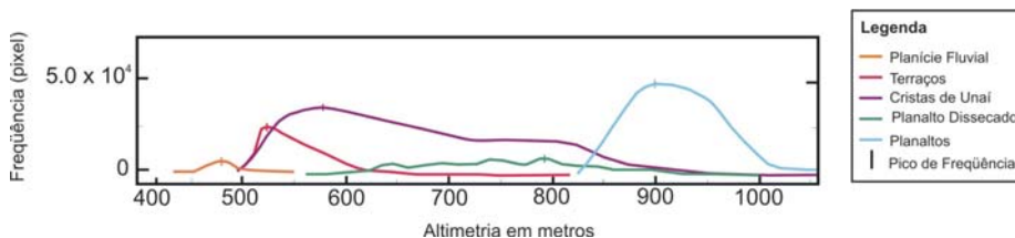
Figura 6 - Análise da frequência de ocorrência das altitudes das unidades geomorfológicas.
