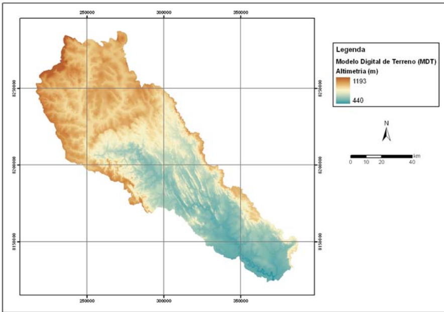
Figura 2 - Modelo Digital de Terreno da bacia do rio Preto.
