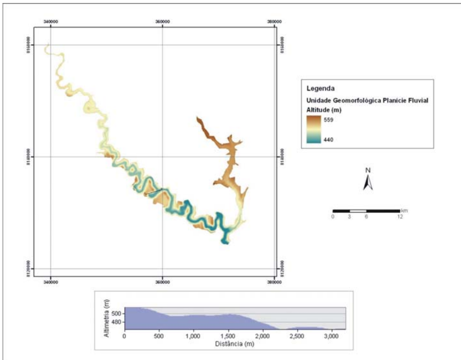
Figura 13 - MDT e perfil da unidade geomorfológica Planície Fluvial.
