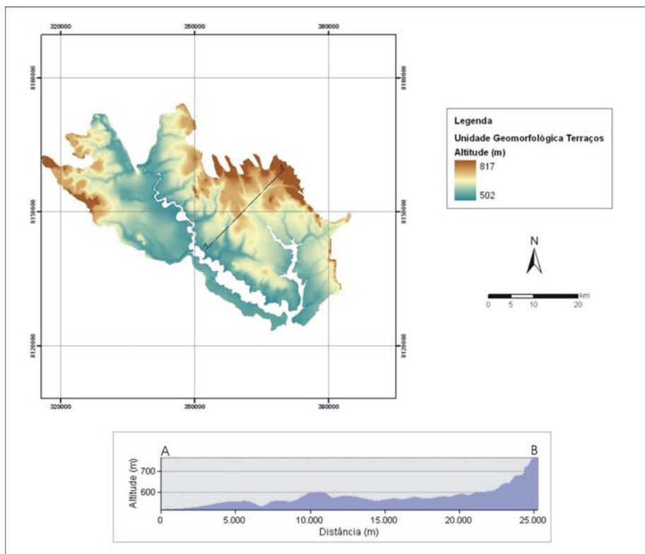
Figura 12 - MDT e perfil topográfico da unidade geomorfológica Terraços.
