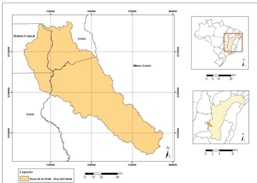
Figura 1 - Localização da bacia do rio Preto.
