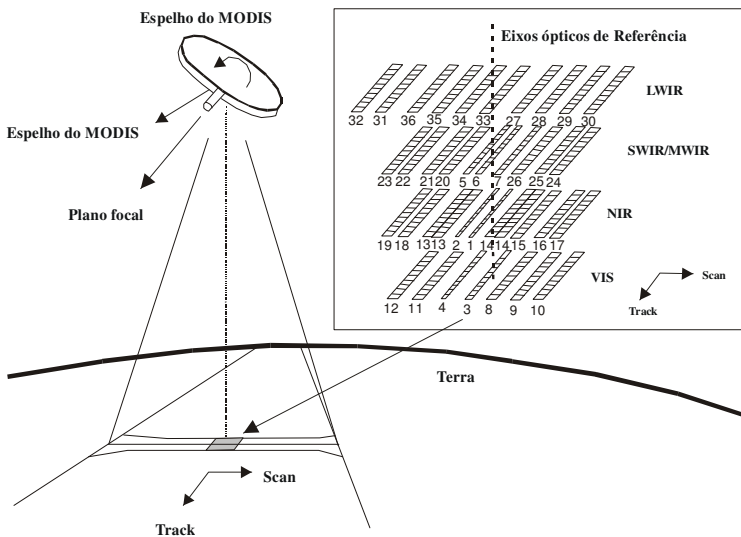
Figura 1 - Apresentação geral da geometria de imageamento do sensor MODIS.
