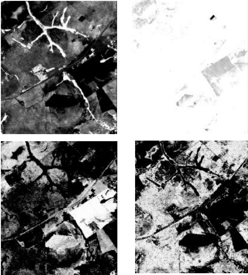
Figura 6 – Imagens classificadas pelo método SCM: (a) vegetação fotossinteticamente ativa, (b) queimada (negativo), (c) vegetação não fotossinteticamente ativa, e (d) solo.
