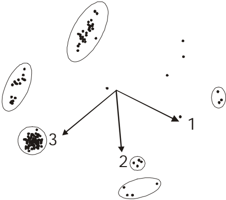
Figura 4 – Visualização dos pixels selecionados como puros num espaço n-dimensional.
