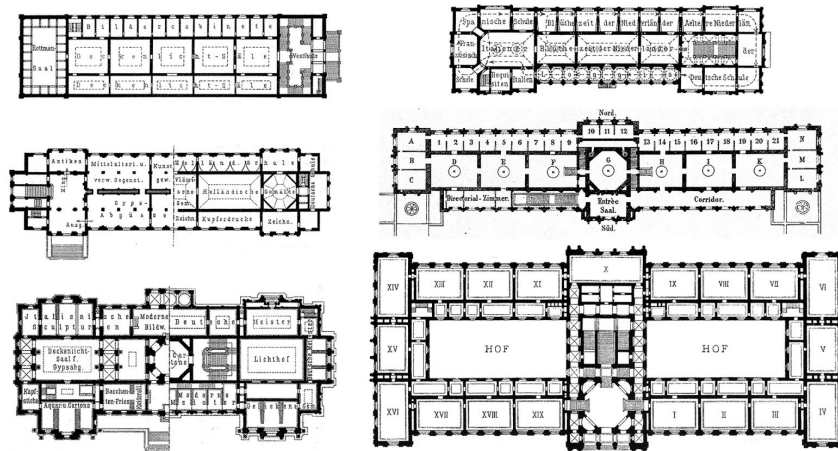
fig. 13 | Piante di musei ottocenteschi. Dall'alto in basso e da sinistra a destra: A. Von Voit, Neue Pinakothek , Monaco di Baviera, 1846-53; H. Dehn-Rothfelser, Gemälde Galerie , Kassel, 1871-77; O. Sommer, Herzog Anton-Ulrich Museum , Braunschweig, 1883-87; G. Semper, Gemäldegalerie , Dresda, 1847-55; L. Lange e H. Licht, Museum der Bildende Kunst , Lipsia, 1885-87; G. Semper e C. von Hasenauer, Kunsthistorisches Museum , Vienna, 1872-89.
