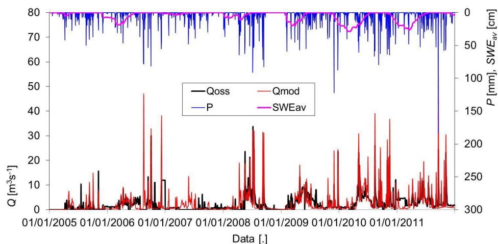
Figura 4. Stazione di Grabiasca, S3. Calibrazione del modello
