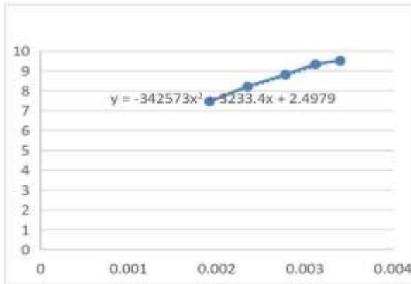
Gambar 3. Uji Stepdrawdown untuk sumur 1.
