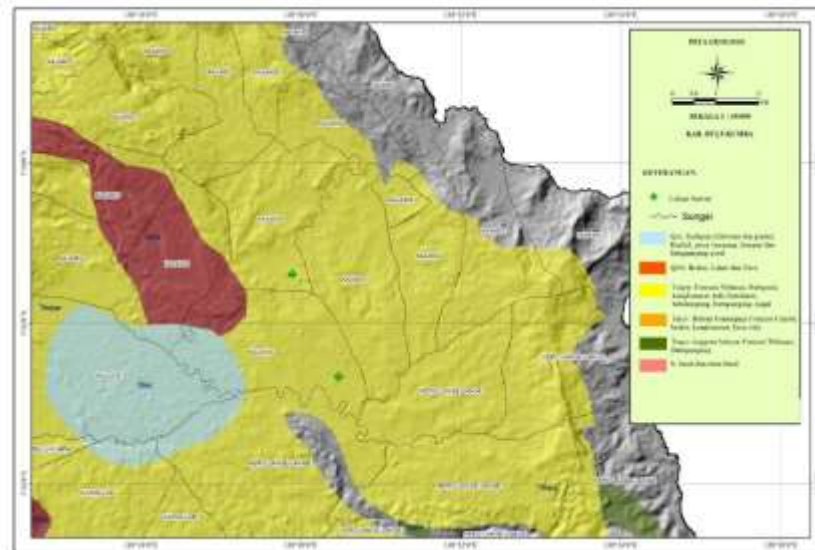
Gambar 1. Peta geologi lokasi penelitian.
