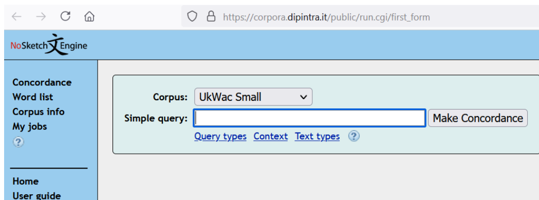
Abbildung 3 Korpuserstellung
