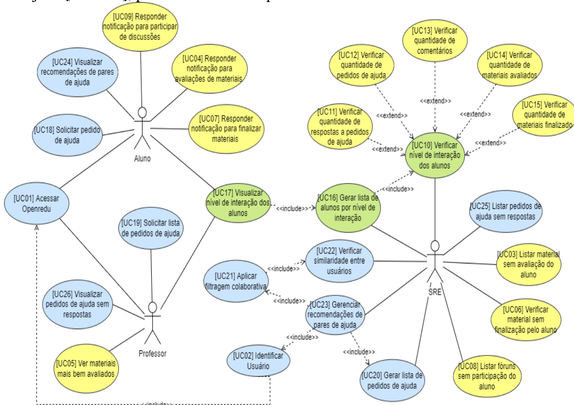
Figura 2 - Casos de Uso para os Atores envolvidos no SRE
