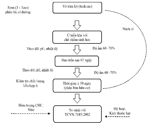
Hình 2: Sơ đồ ủ phân bón vỏ tôm lột
