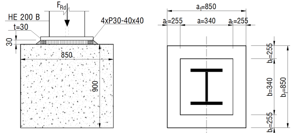
Hình 2: Cấu tạo chi tiết chân cột
