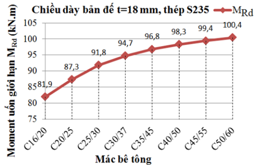
Hình 9: Biểu đồ quan hệ giữa moment chịu uốn giới hạn M_{Rd} với từng loại mác bê tông
