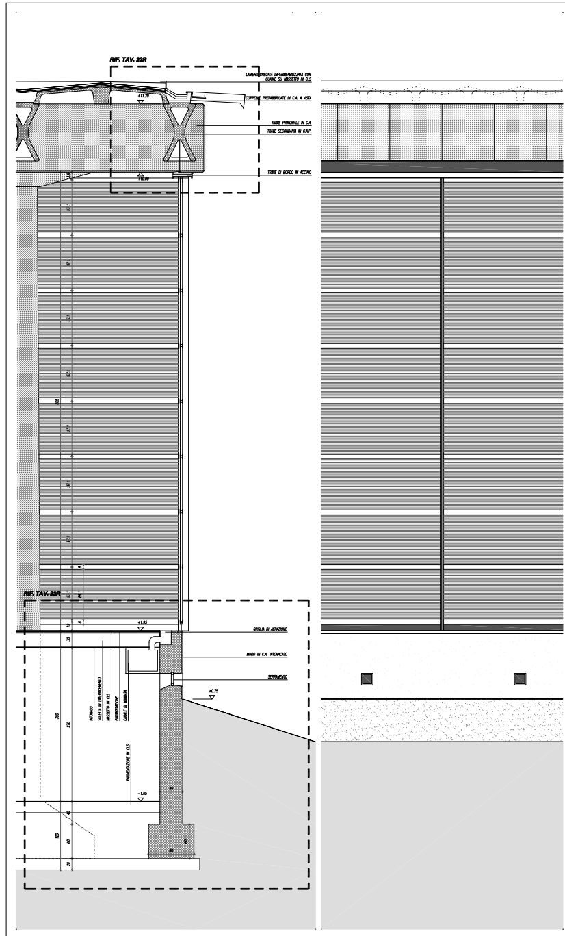
05 | Sezione verticale del progetto della chiesa dove si nota l'aggancio dei montanti in acciaio Section top-bottom of the steel facade system
