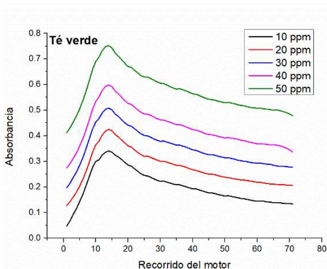
Figura 5. Curva de respuesta espectral para los complejos de té verde-Fe 3+ (diferentes concentraciones) obtenidos con el prototipo, después de un suavizado.
