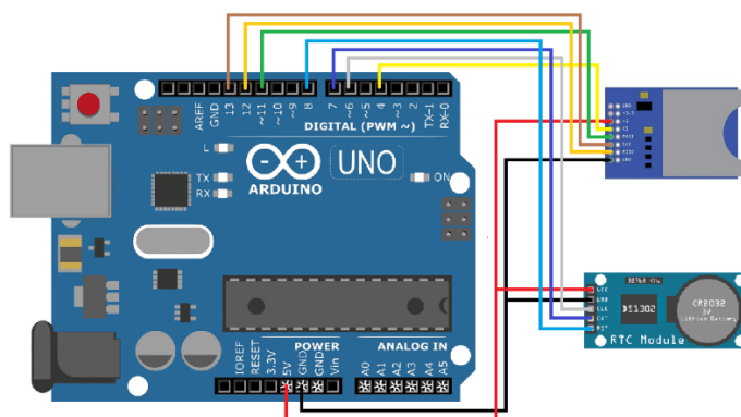
Figura 1 – Esquema de ligação dos Shields na placa Arduino
