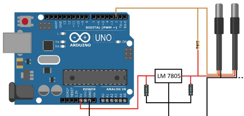
Figura 2 – Esquema de ligação dos sensores de temperatura DS18B20 na placa Arduino.
