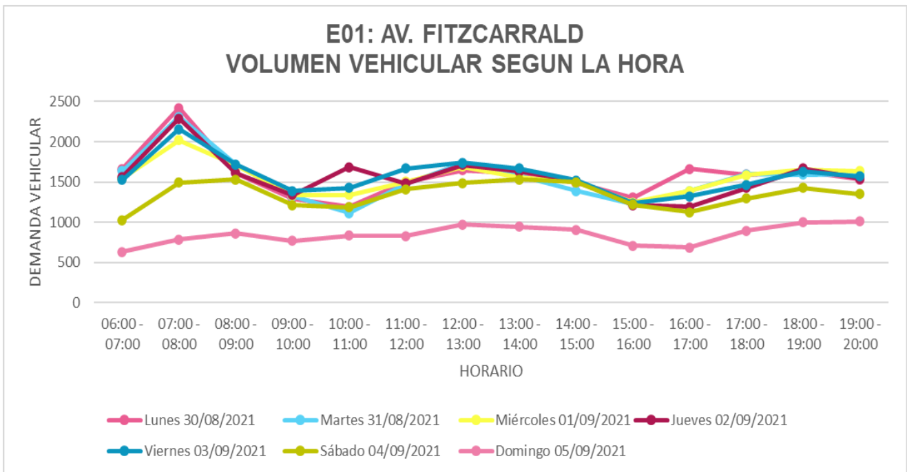
Gráfico 2: Demanda vehicular de la estación 01
