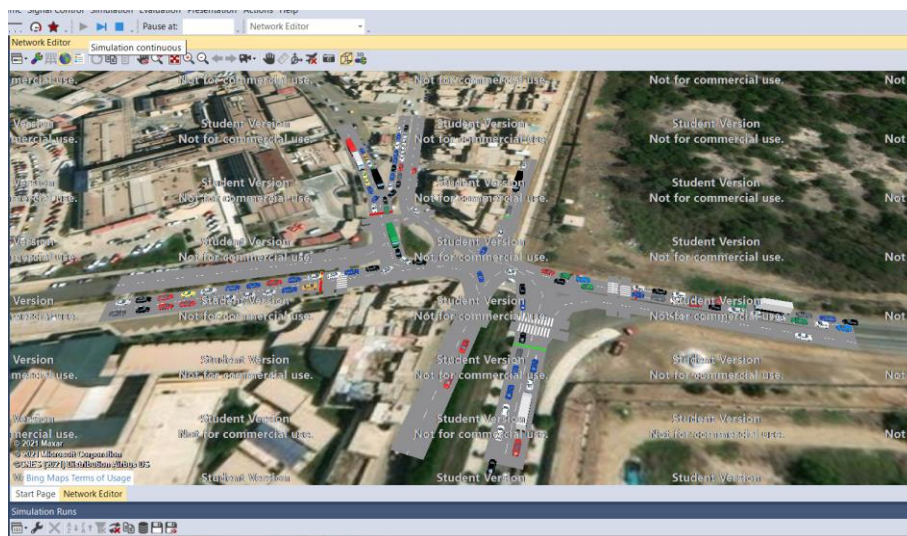
Ilustración 36: simulación de flujo vehicular de la situación actual de la zona de estudio.
