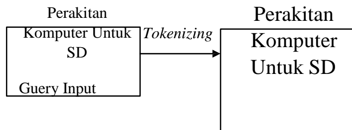
Gambar 3 Tahapan Tokenizing
