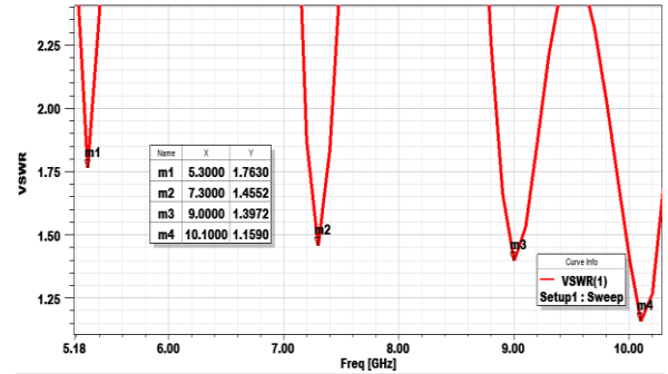
Fig.10. VSWR
