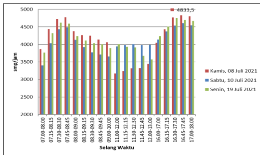
Gambar 4. Arus Lalu Lintas (Smp/jam) Simpang Selama 3 hari Survei pada Jam-jam Sibuk
