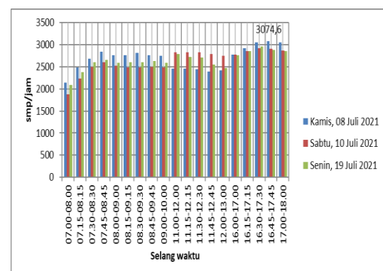
Gambar 7 Data Arus Lalu Lintas Simpang Bersinyal
