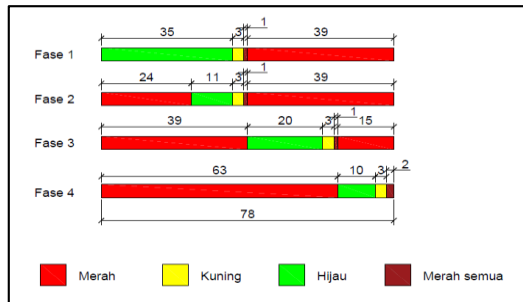
Gambar 8 Waktu Siklus Simpang Bersinyal
