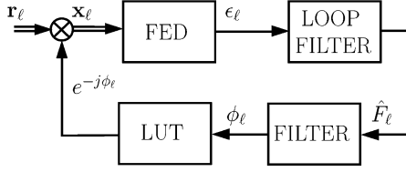
Fig. 4. AFC scheme.
