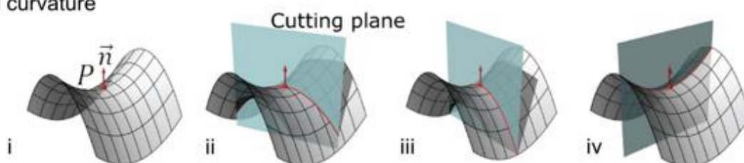
b. normal curvature
