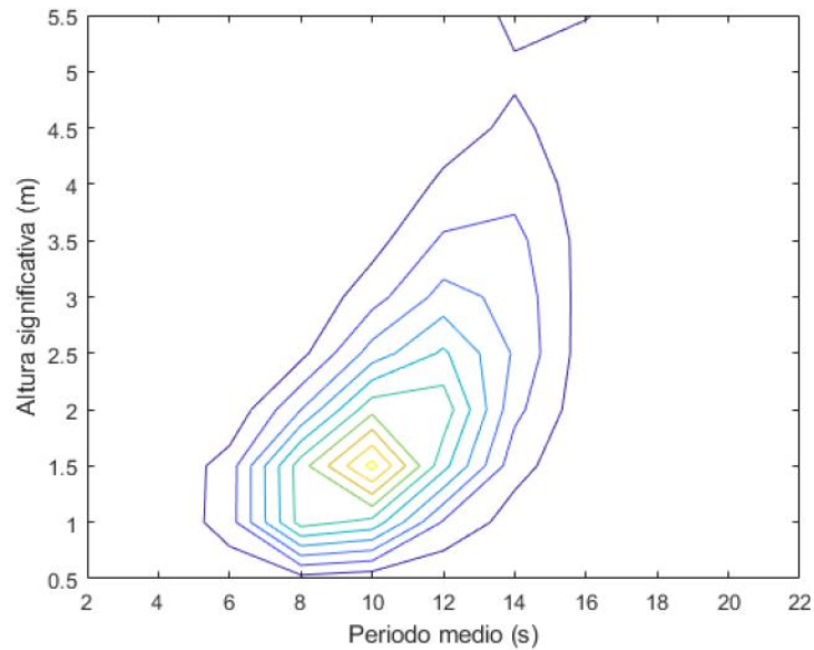
Figura 32. Porcentaje de oleaje característico de la zona.
