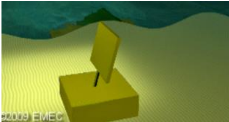
Figura 27. Mecanismo OWSC.
