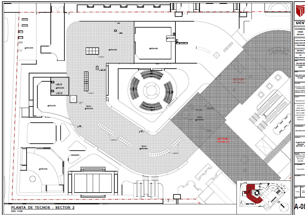
Planta de Techos - Sector 2 (Esc. 1:125)
