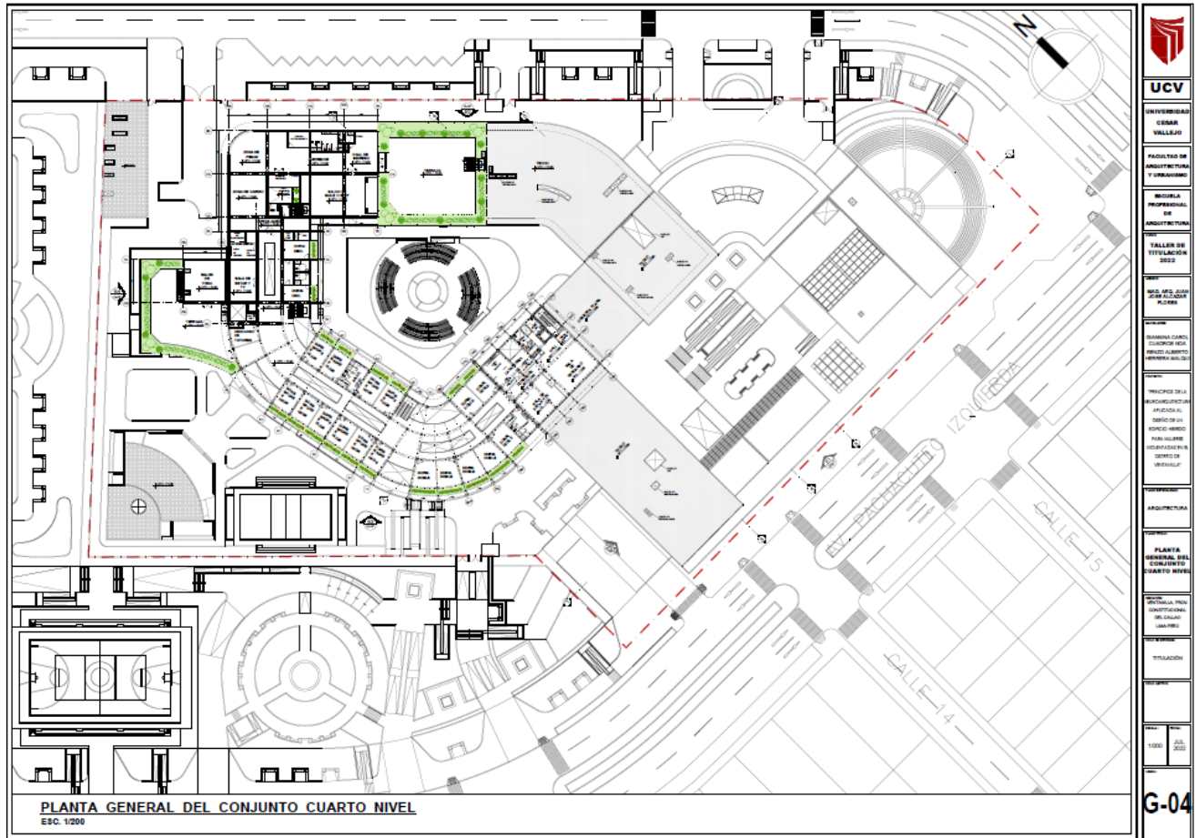
Planta General Cuarto Nivel - Esc. 1/200
