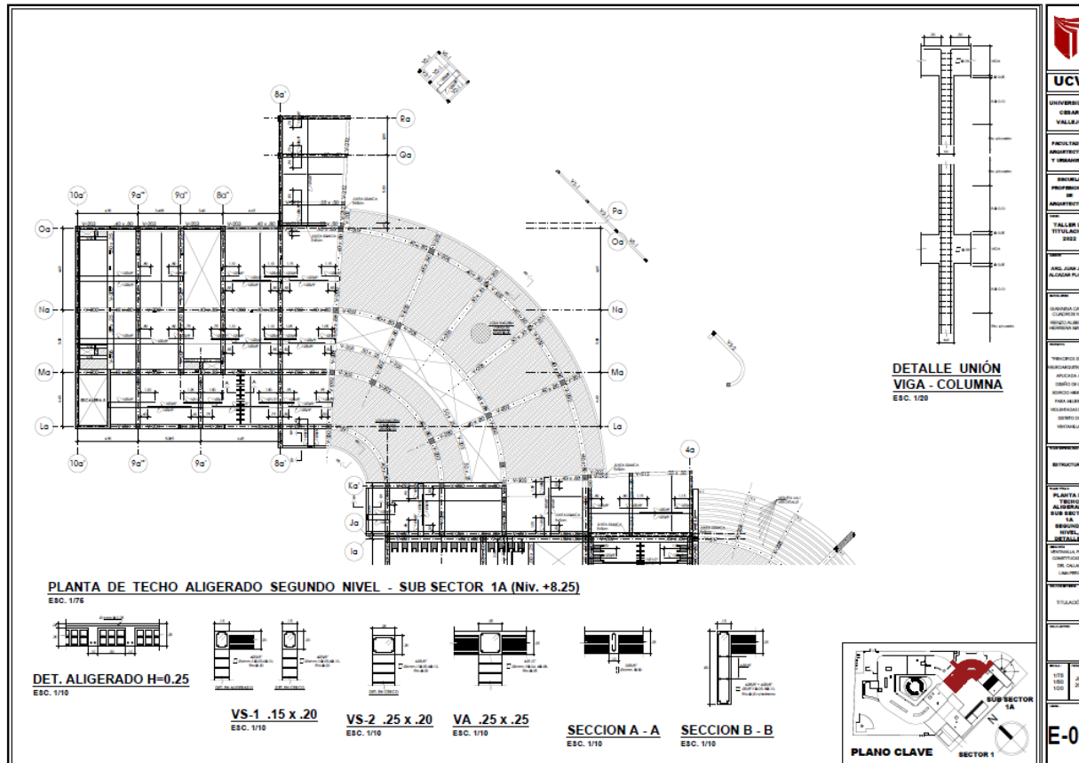
Planta de Techo Aligerado Segundo Nivel – Sub Sector 1A
