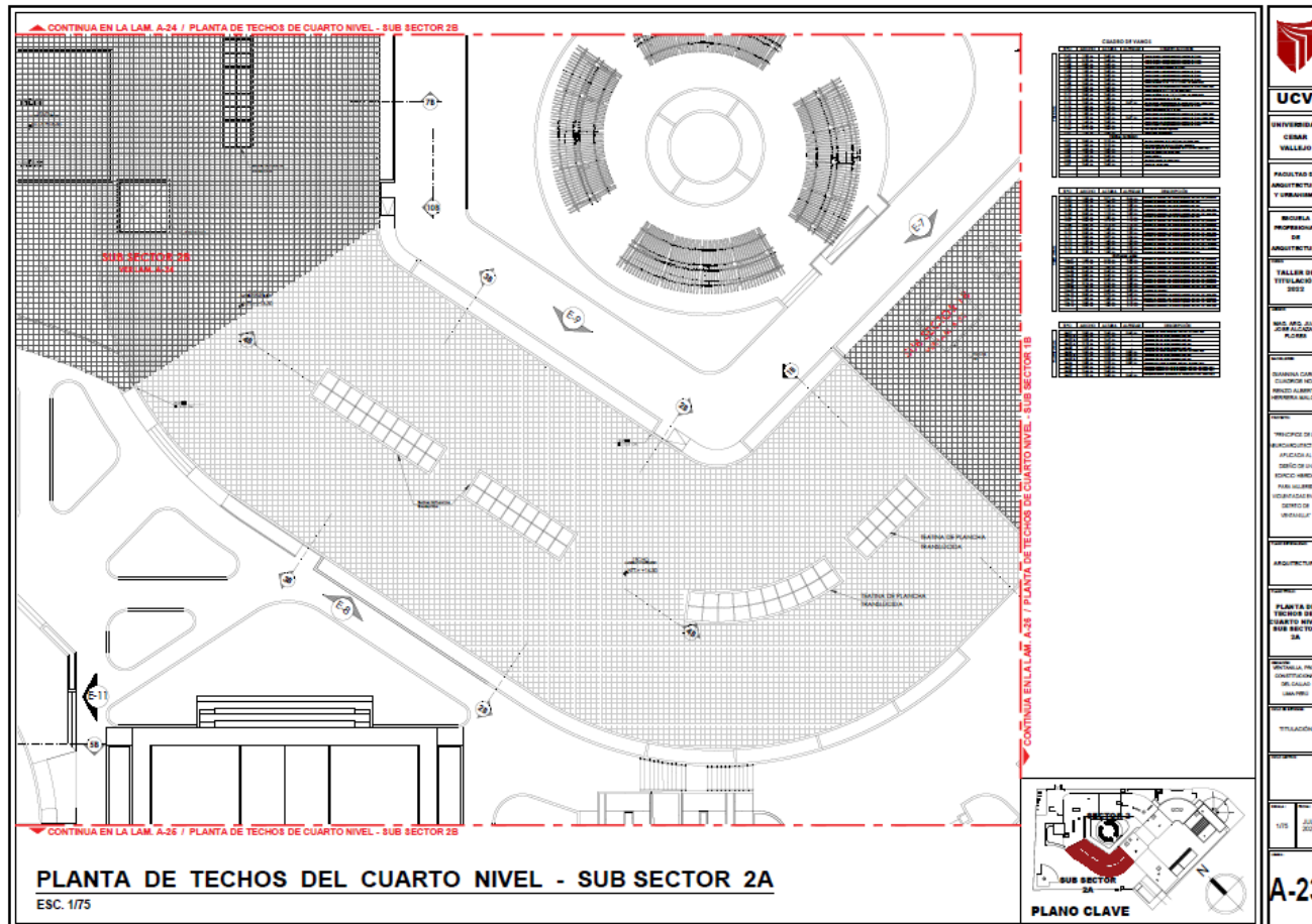
Planta de Techos del Cuarto Nivel – Sub Sector 2A (Esc. 1:75)
