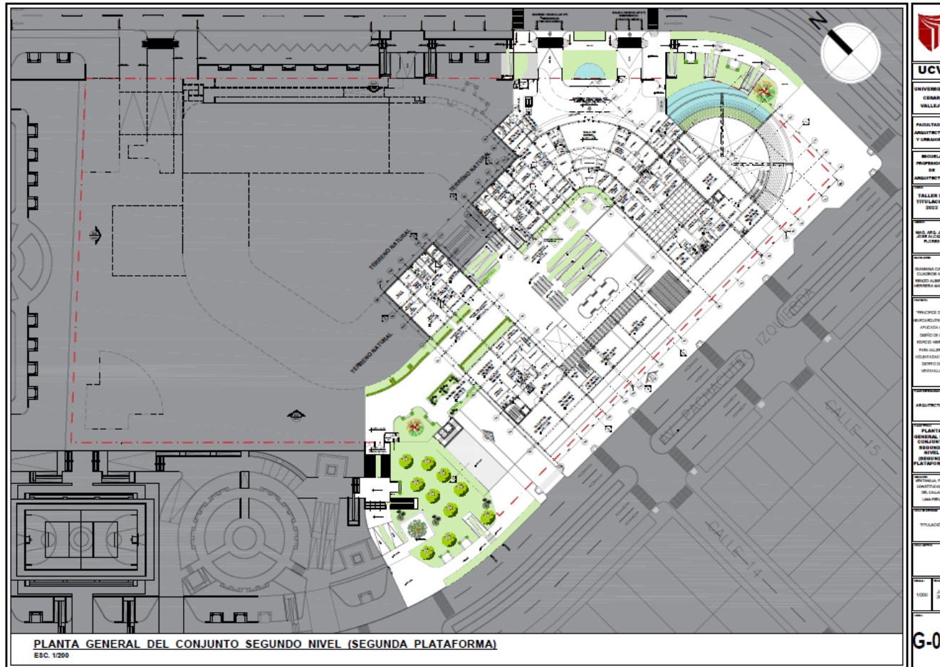
Planta General Segundo Nivel - Esc. 1/200
