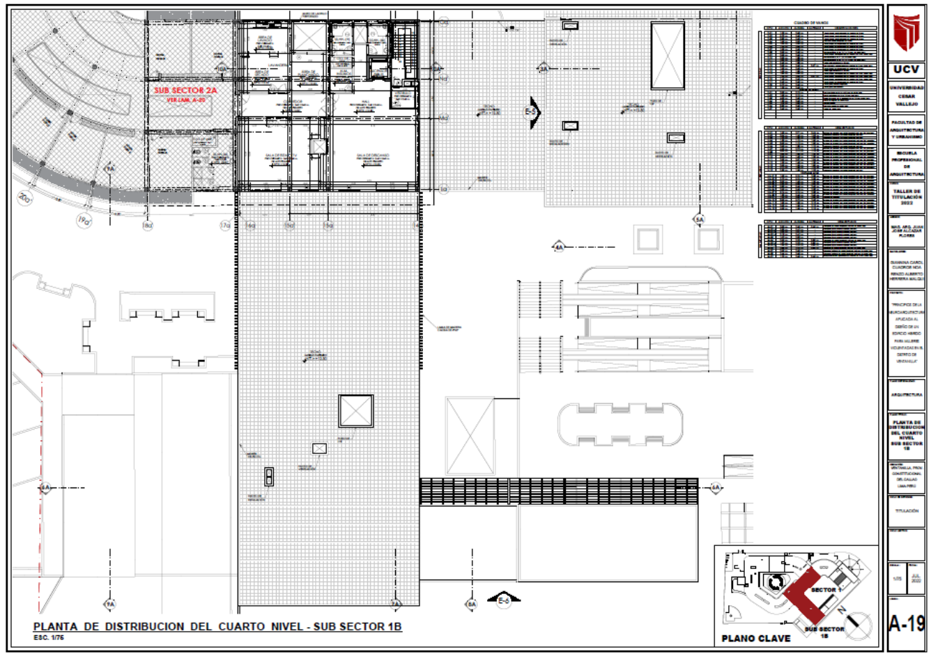
Planta de Distribución de Cuarto Nivel - Sub Sector 1B (Esc.1:75)
