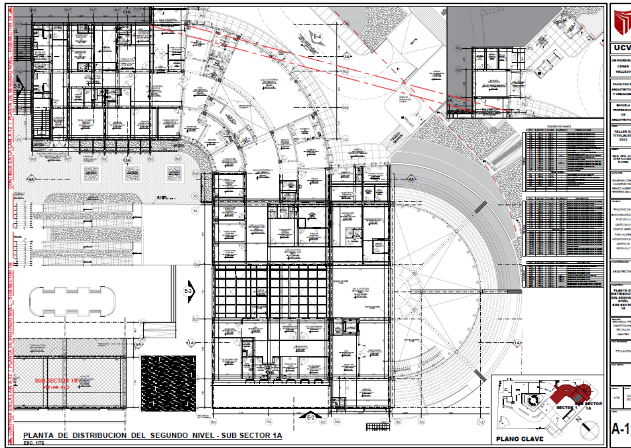
Planta de Distribución del Segundo Nivel - Sub Sector 1A (Esc. 1:75)
