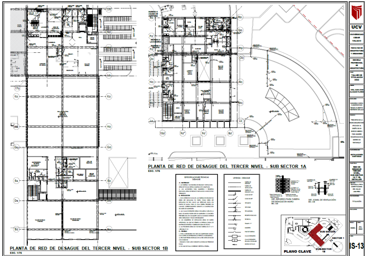
Planta de Red de Desagüe del Tercer Nivel – Sub Sector 1 A y 1 B
