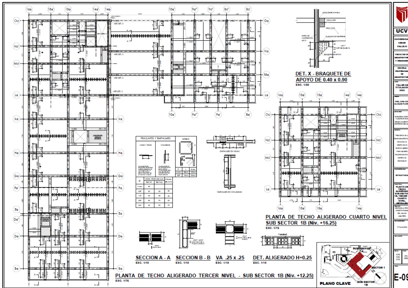
Planta de Techo Aligerado Tercer Nivel – Sub Sector 1B
