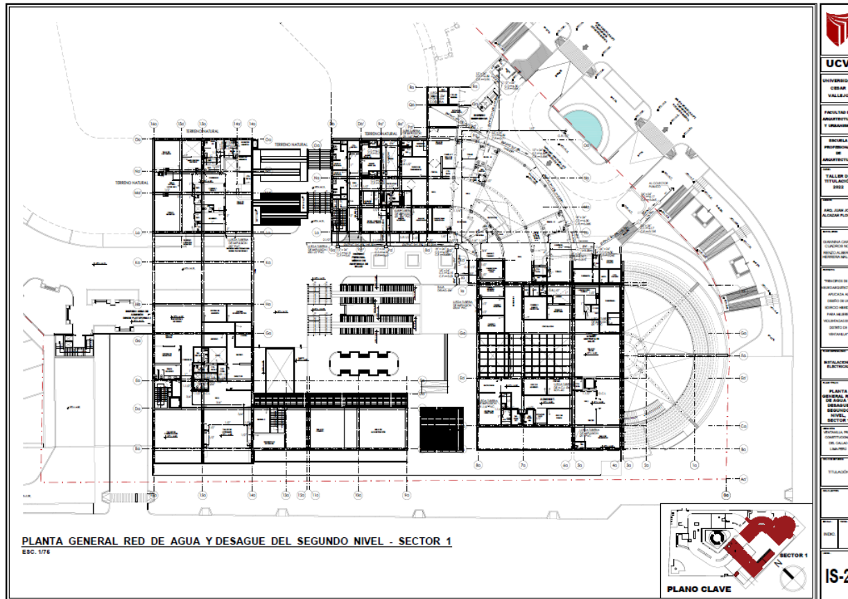
Planta General Red de Agua y Desagüe del Segundo Nivel – Sector 1
