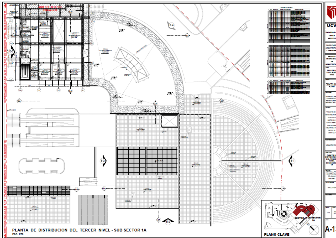
Planta de Distribución del Tercer Nivel - Sub Sector 1A (Esc. 1:75)
