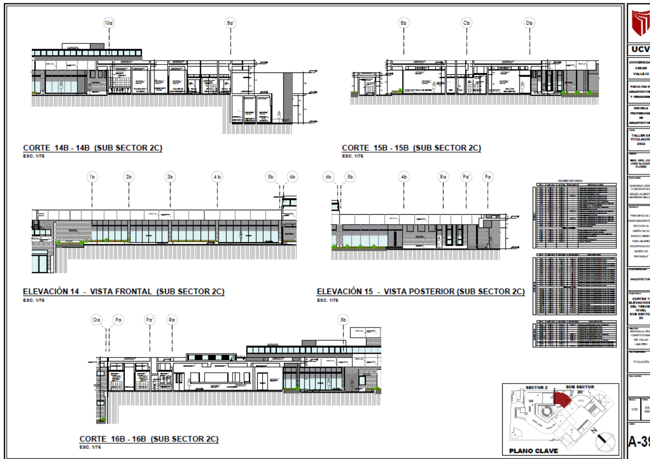
Plano de Corte y Elevación – Sub Sector 2C
