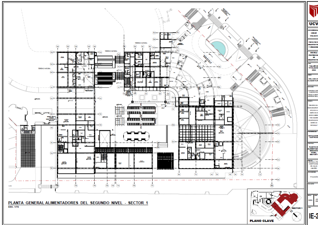
Planta General Alimentadores del Segundo Nivel –Sector 1
