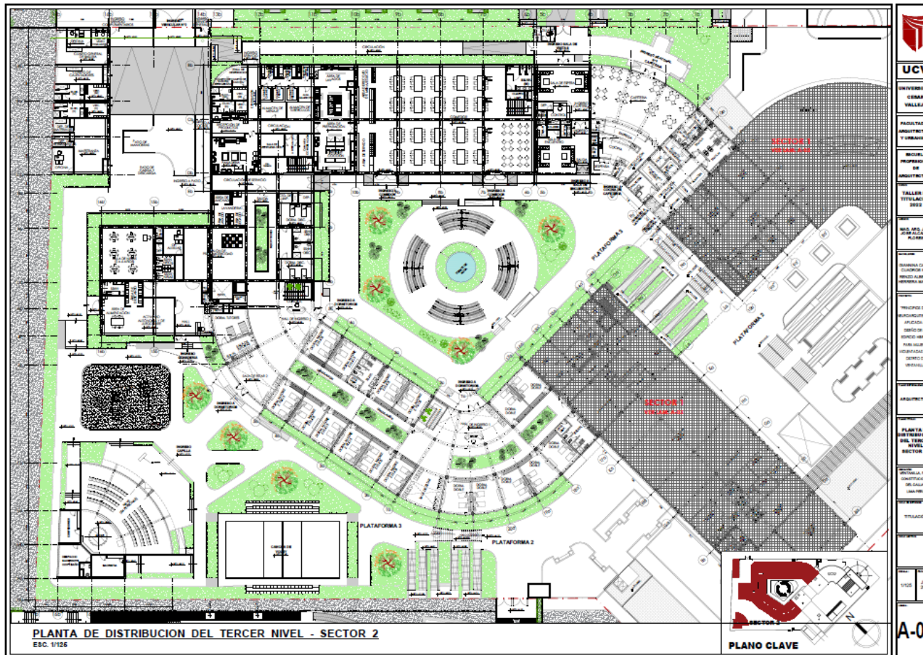
Planta de Distribución del Tercer Nivel - Sector 2 (Esc. 1:125)
