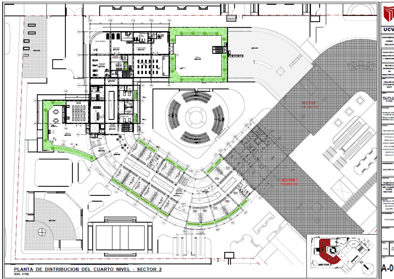
Planta de Distribución del Cuarto Nivel - Sector 2 (Esc. 1:125)
