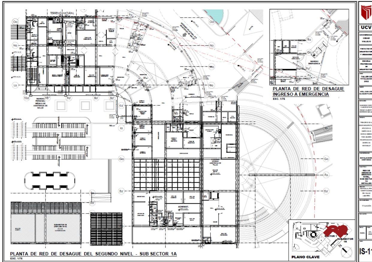
Planta de Red de Desagüe del Segundo Nivel – Sub Sector 1A
