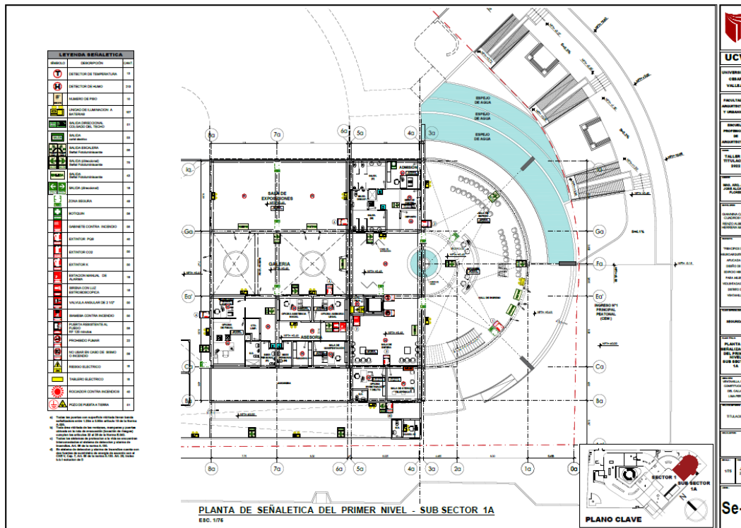
Plano de Señalética del Primer Nivel – Sub Sector 1A
