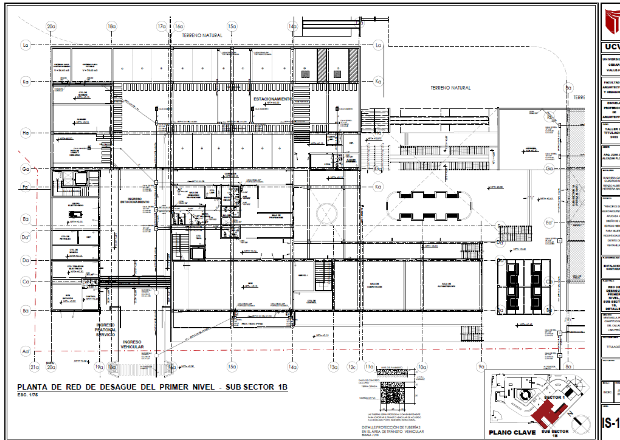
Planta de Red de Desagüe del Primer Nivel – Sub Sector 1B
