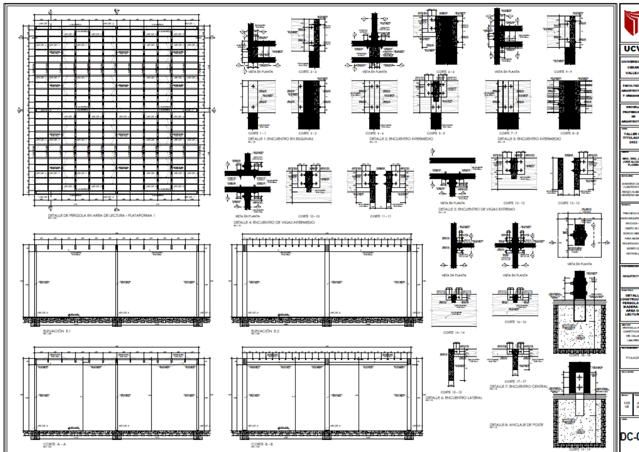
Detalle de Pérgola - Área de Lectura
