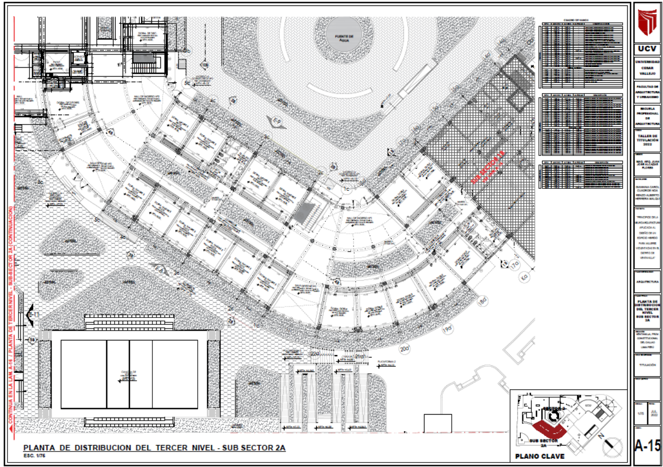
Planta de Distribución del Tercer Nivel - Sub Sector 2A (Esc.1:75)
