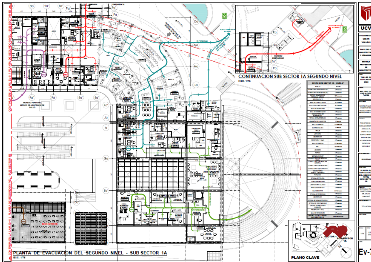
Plano de Evacuación del Segundo Nivel – Sub Sector 1A
