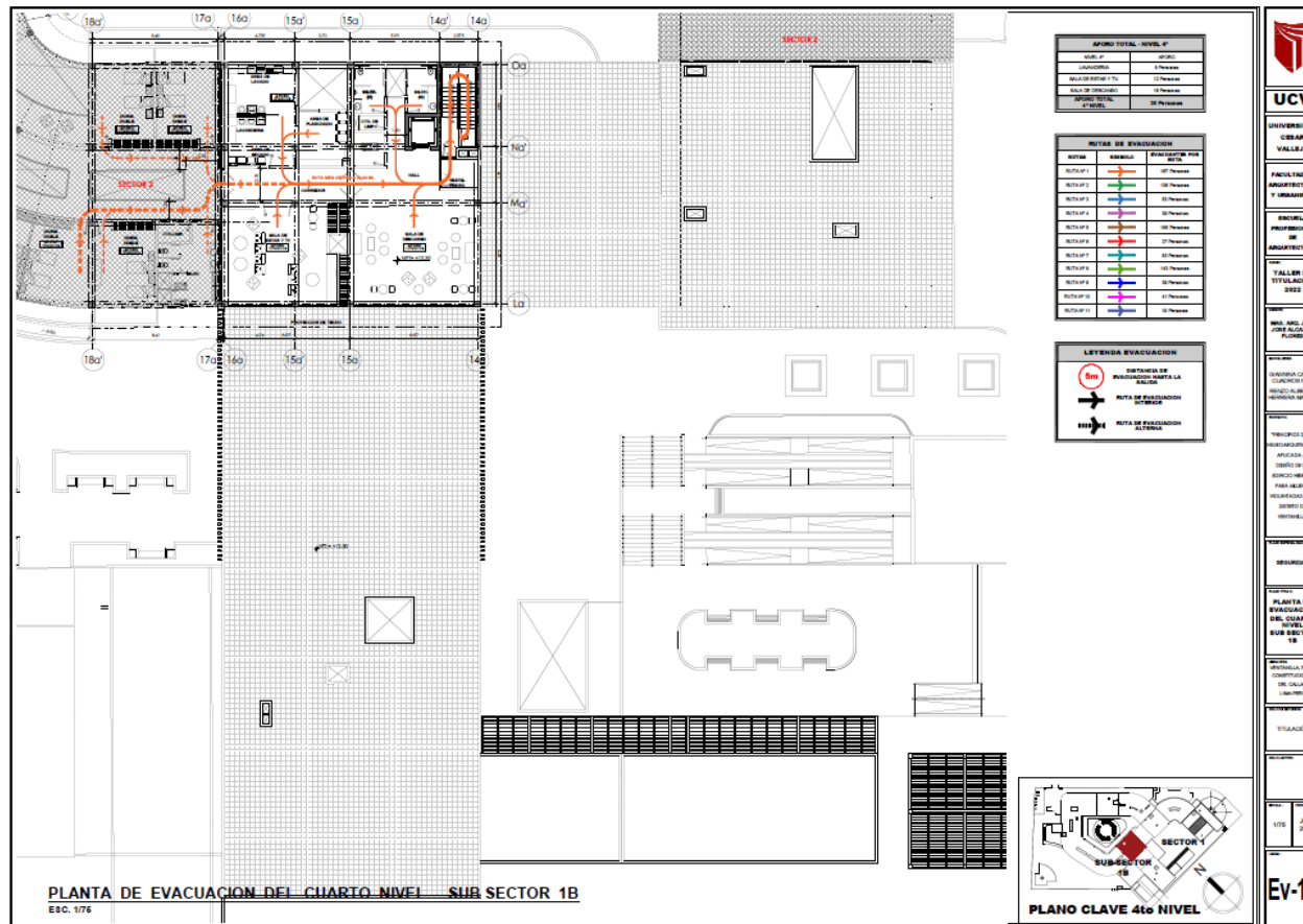
Plano de Evacuación del Cuarto Nivel - Sub Sector 1B
