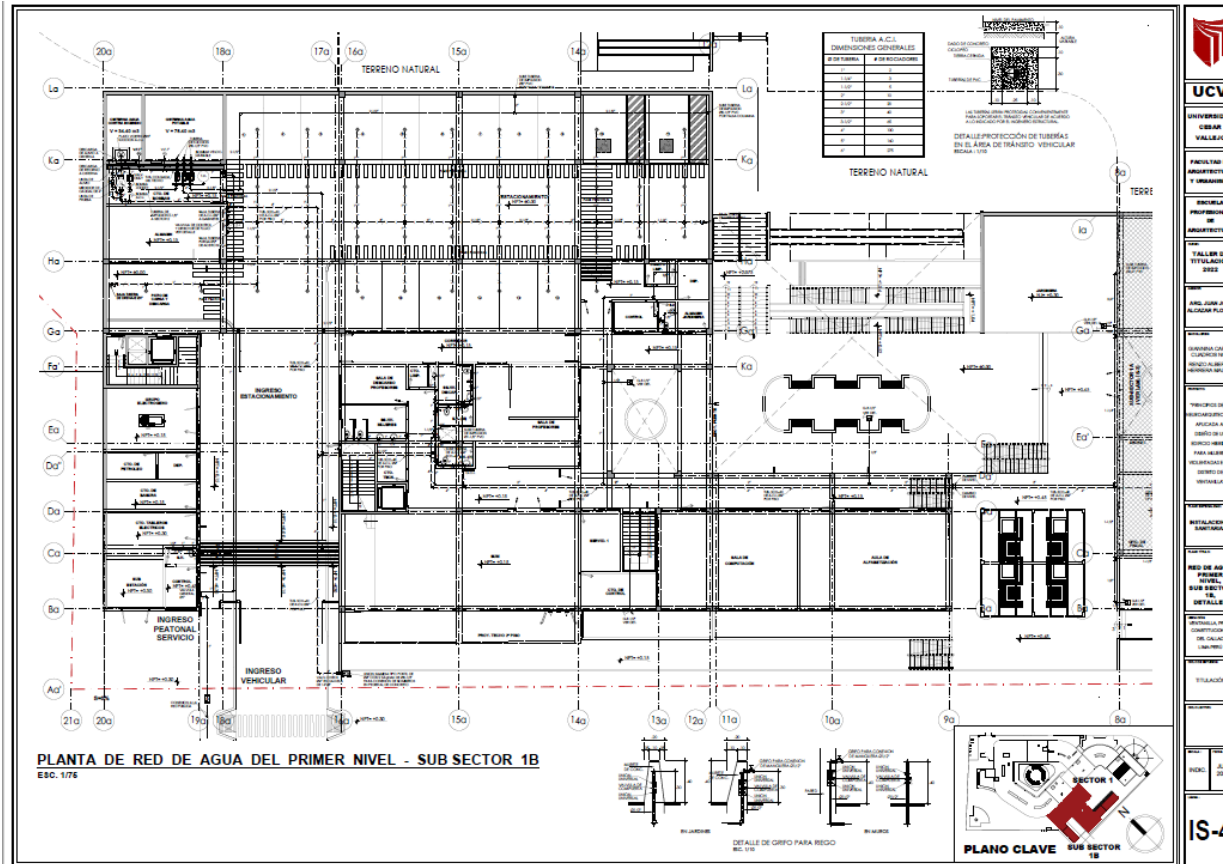
Planta de Red de Agua del Primer Nivel – Sub Sector 1B
