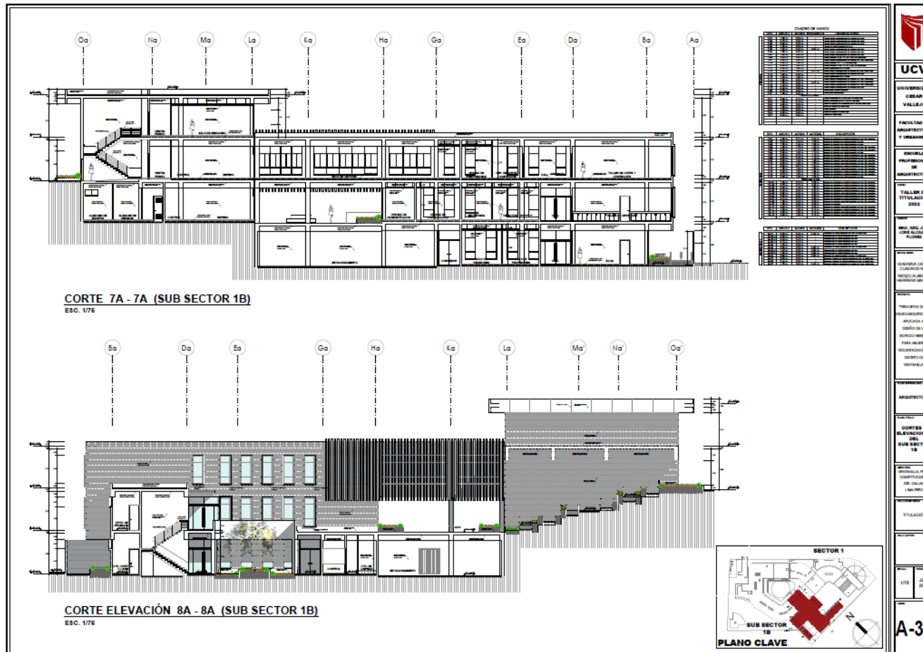
Plano de Corte y Elevación – Sub Sector 1B
