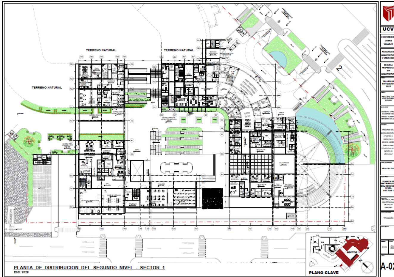
Planta de Distribución del Segundo Nivel - Sector 1 (Esc. 1:125)
