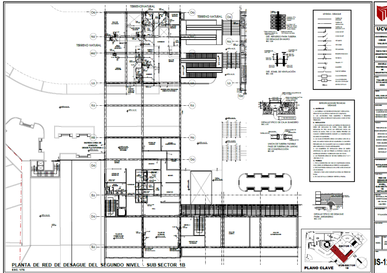
Planta de Red de Desagüe del Segundo Nivel – Sub Sector 1B
