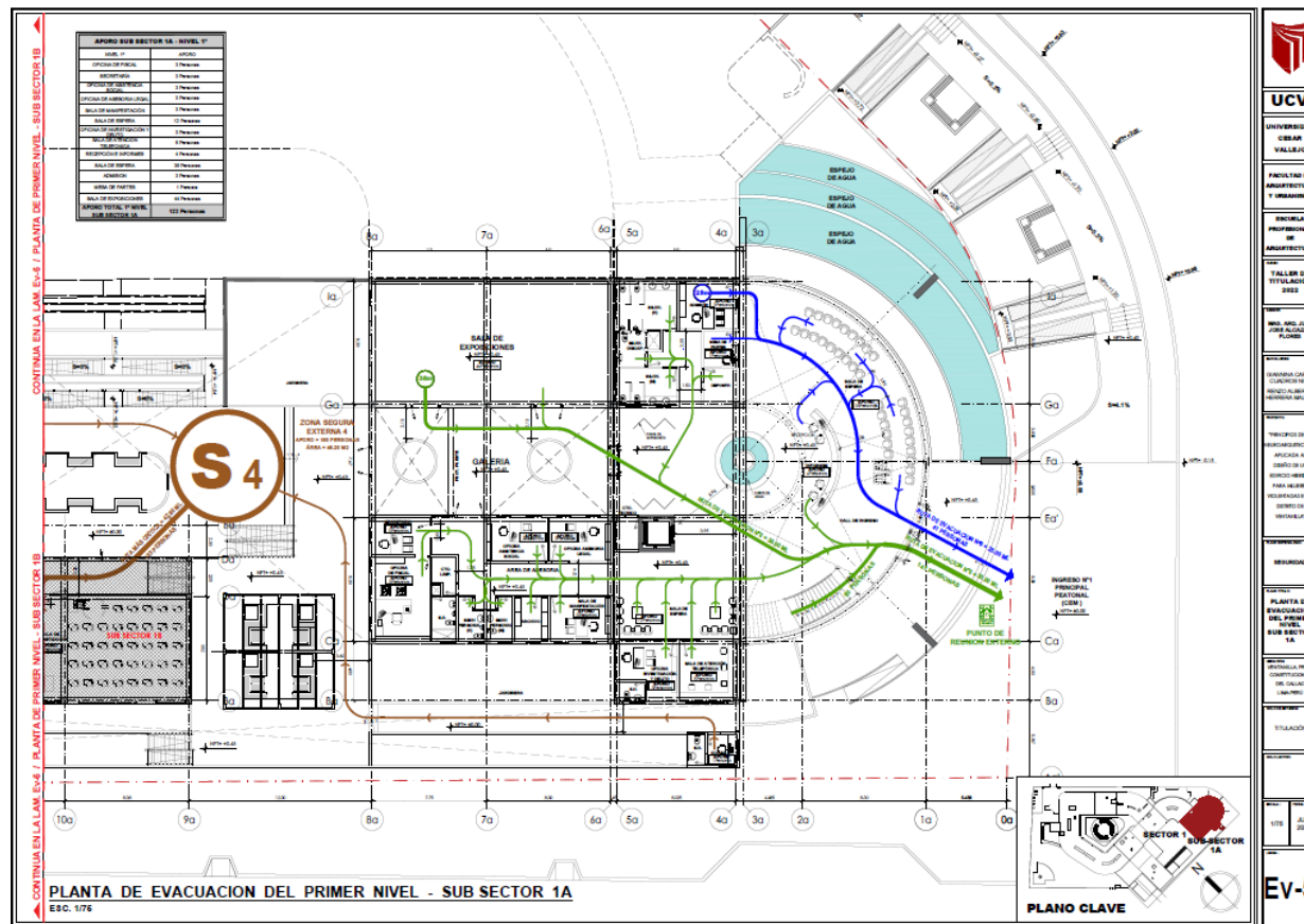
Plano de Evacuación del Primer Nivel – Sub Sector 1A
