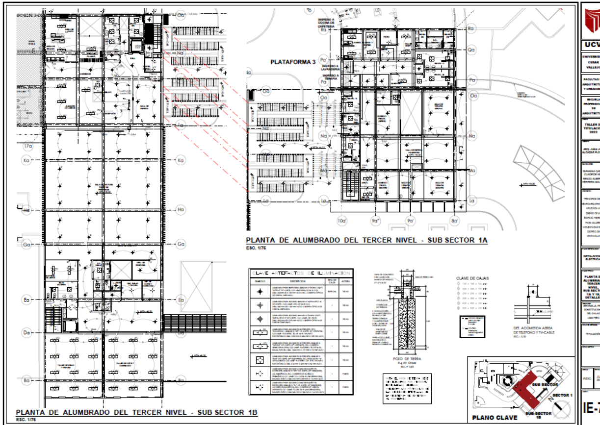
Planta de Alumbrado del Tercer Nivel – Sub Sector 1 A Y 1 B
