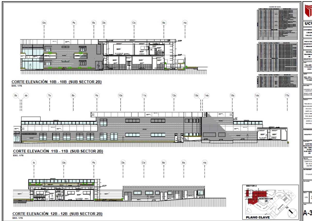
Plano de Corte y Elevación – Sub Sector 2B
