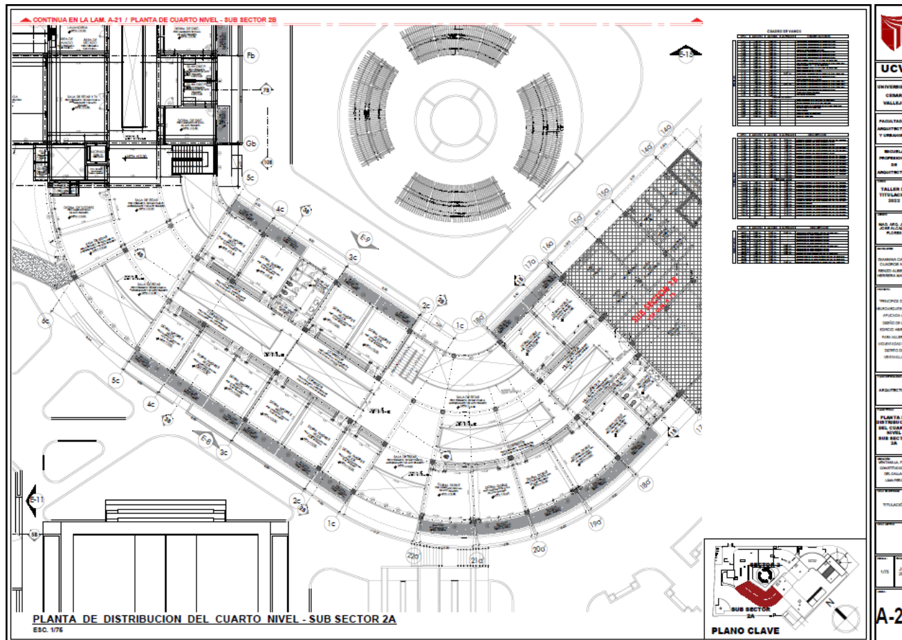
Planta de Distribución del Cuarto Nivel - Sub Sector 2A (Esc. 1:75)
