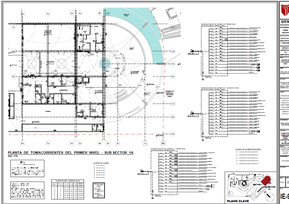
Planta de Tomacorrientes del Primer Nivel – Sub Sector 1A
