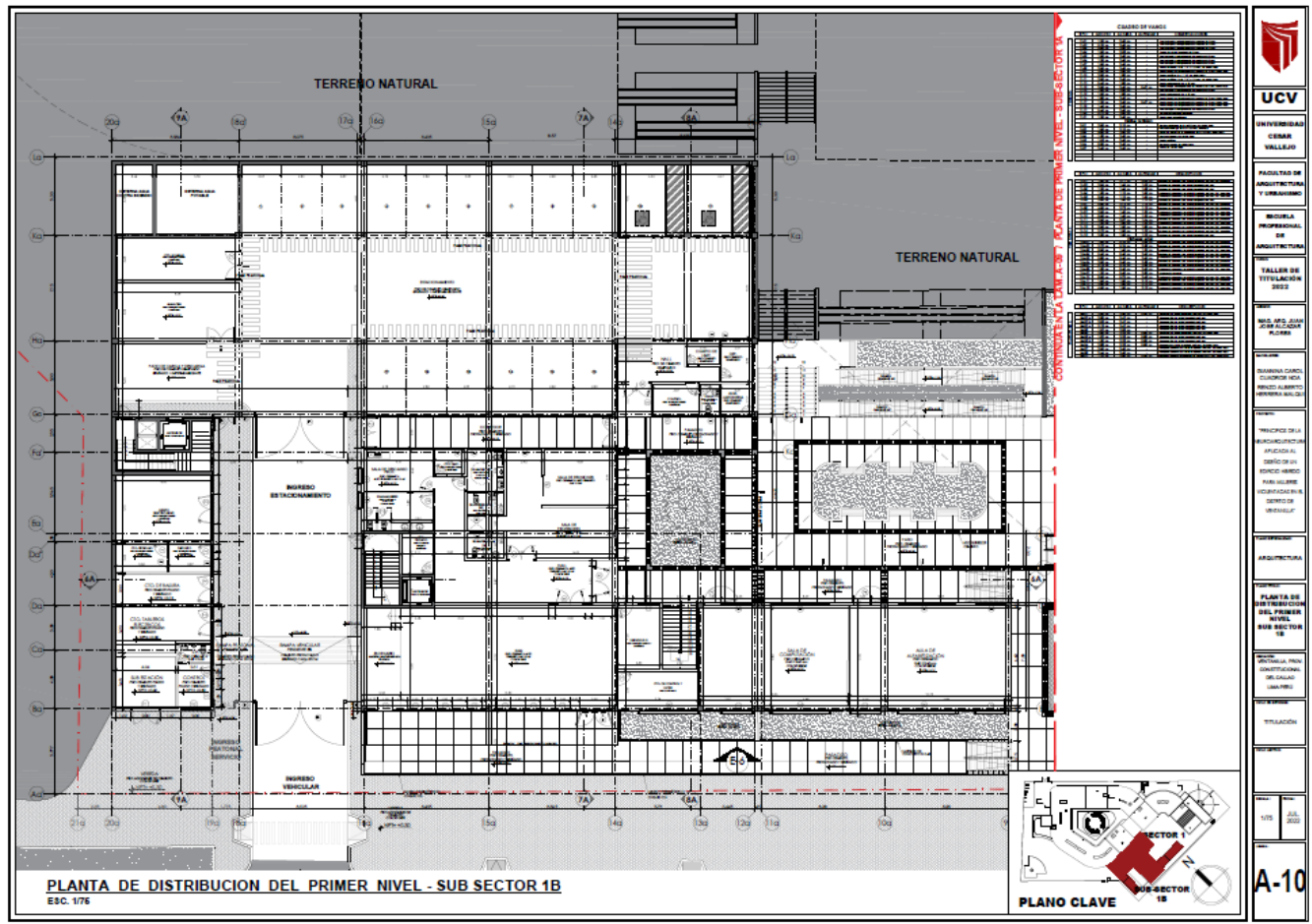
Planta de Distribución del Primer Nivel - Sub Sector 1B (Esc. 1:75)
