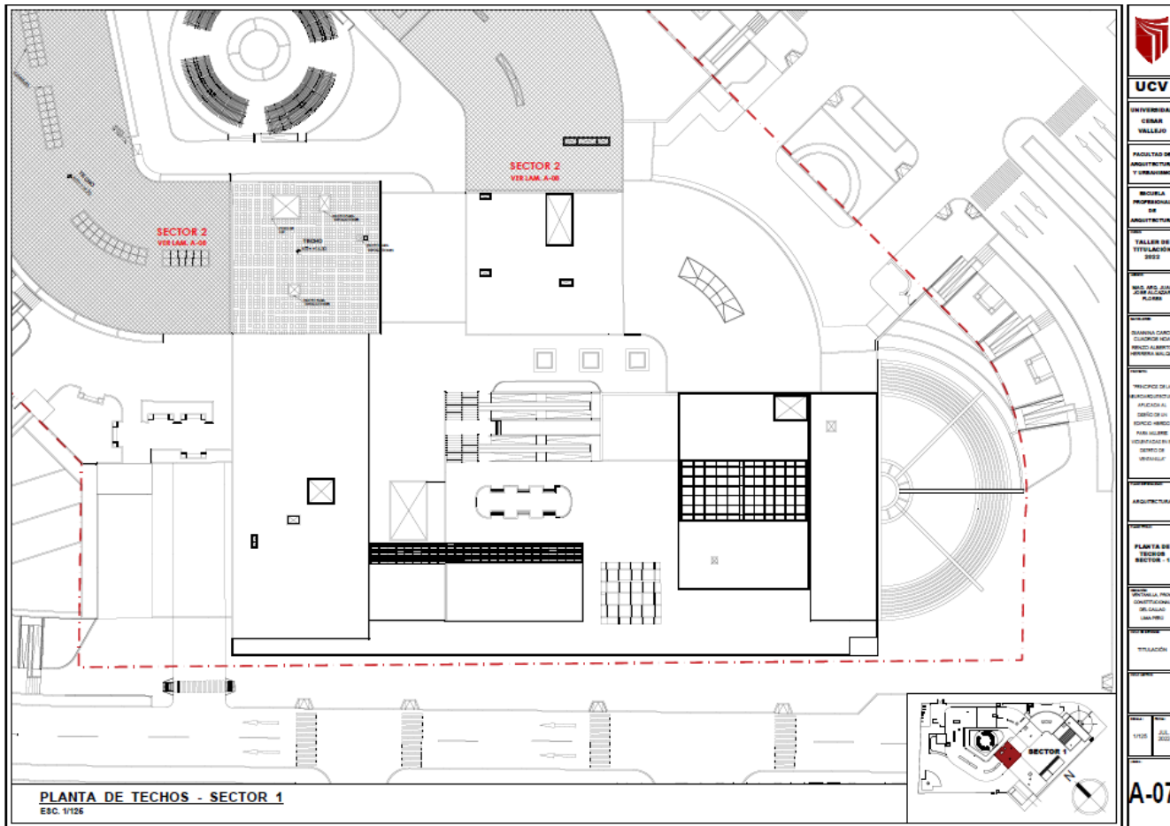
Planta de Techos - Sector 1 (Esc. 1:125)
