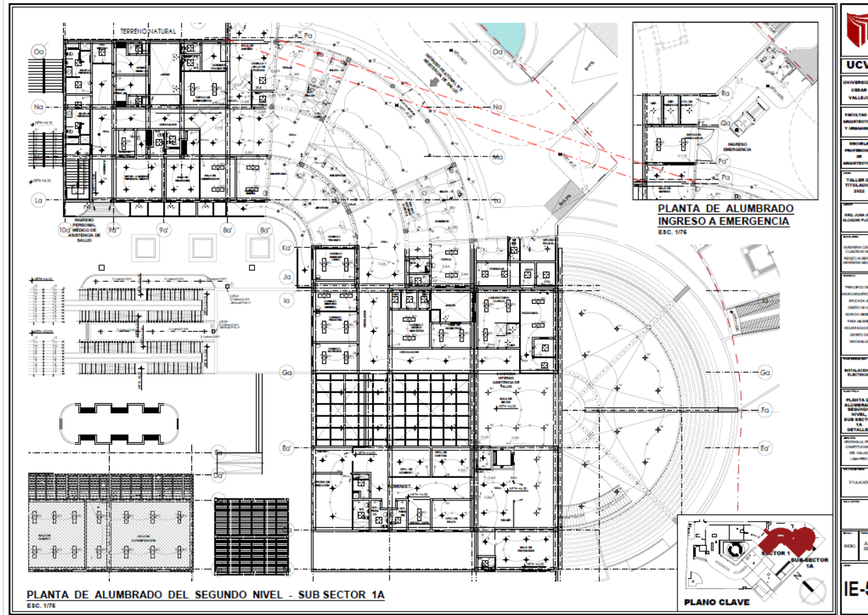
Planta de Alumbrado del Segundo Nivel – Sub Sector 1A
