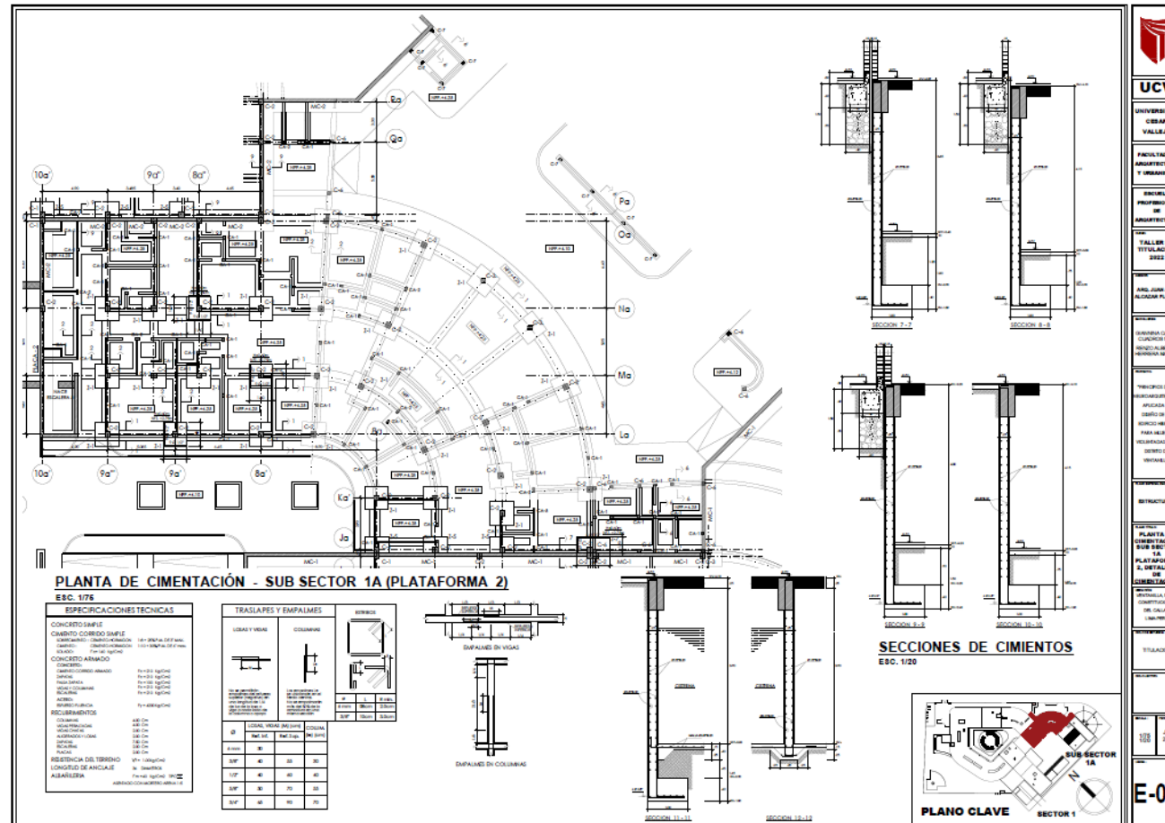
Plano de Cimentación – Sub Sector 1A
