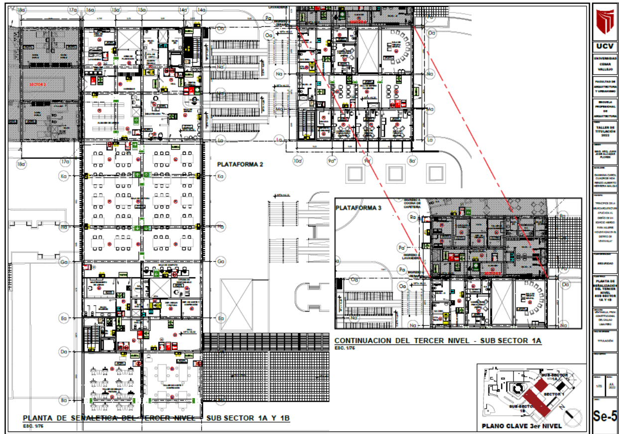
Plano de Señalética del Tercer Nivel – Sub Sector 1A y 1B
