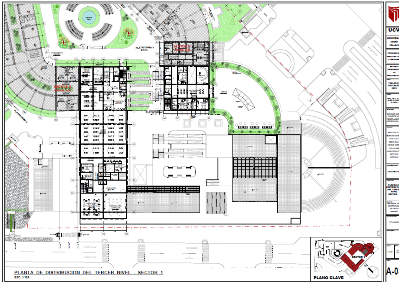
Planta de Distribución del Tercer Nivel - Sector 1 (Esc. 1:125)
