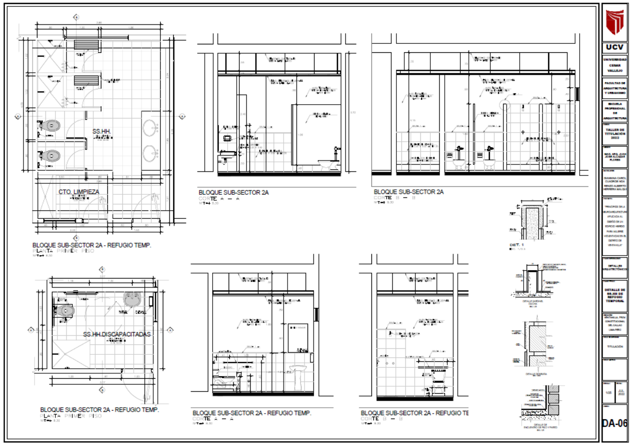
Detalle de Servicios Higiénicos de Refugio Temporal
