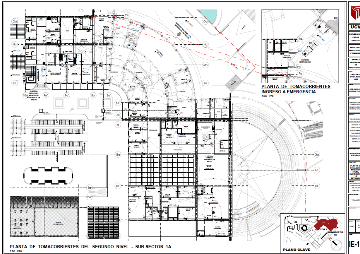
Planta de Tomacorrientes del Segundo Nivel – Sub Sector 1A
