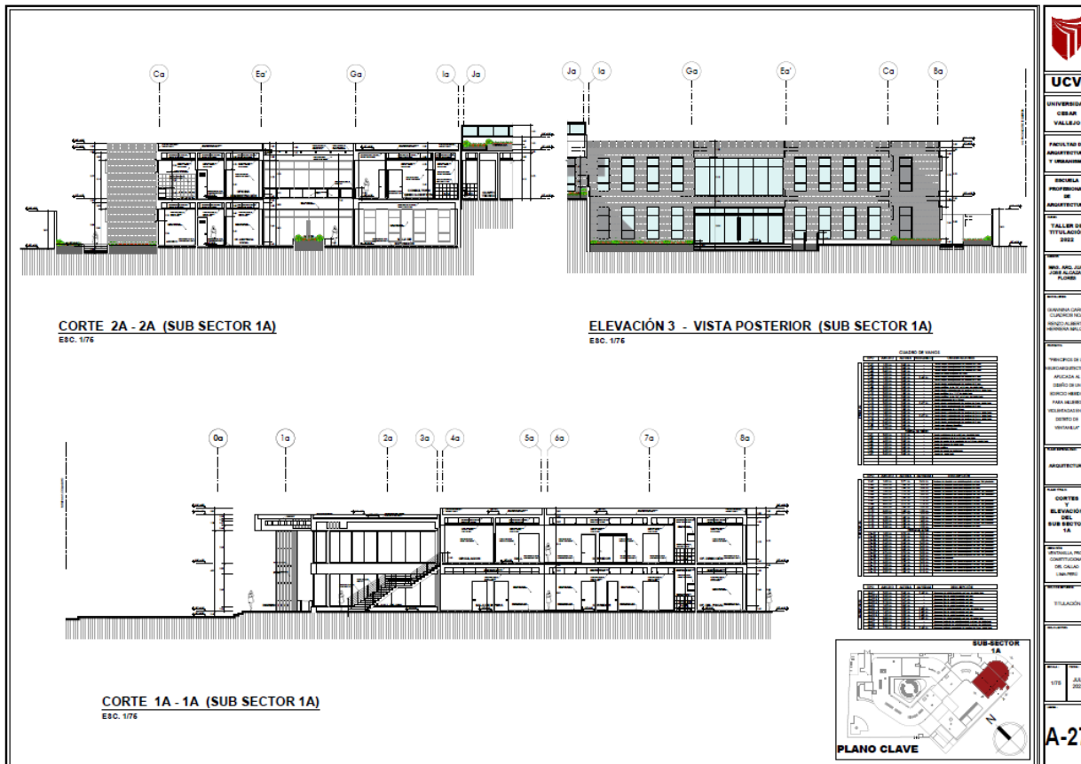
Planos de Cortes y Elevaciones – Sub Sector 1A
