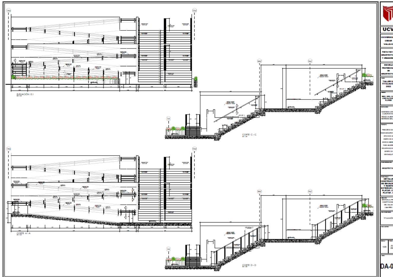
Corte y Elevación de Escalera y Rampa Exterior (Plataforma 2 a Plataforma 3)
