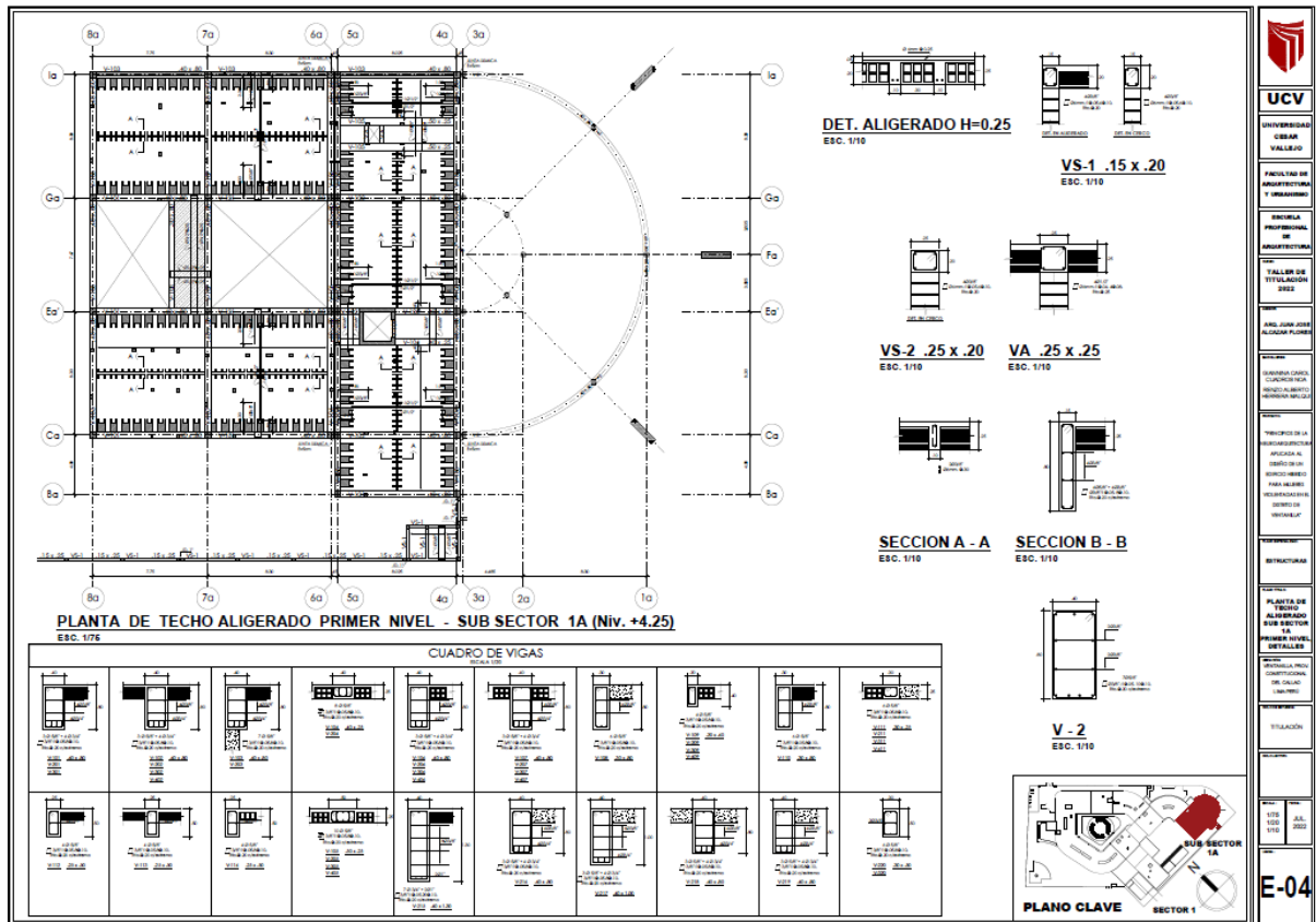
Planta de Techo Aligerado Primer Nivel – Sub Sector 1A
