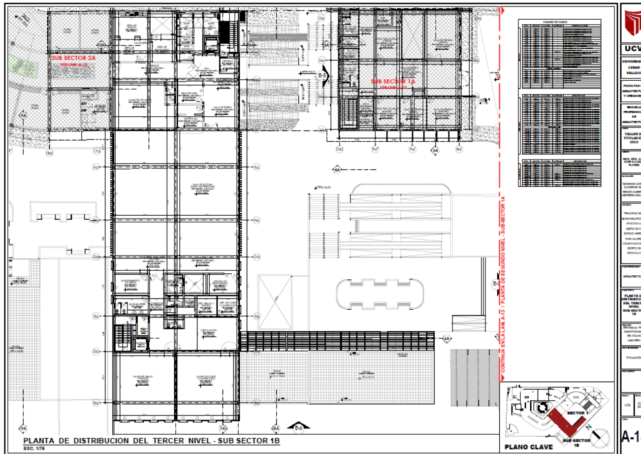
Planta de Distribución del Tercer Nivel - Sub Sector 1B (Esc. 1:75)
