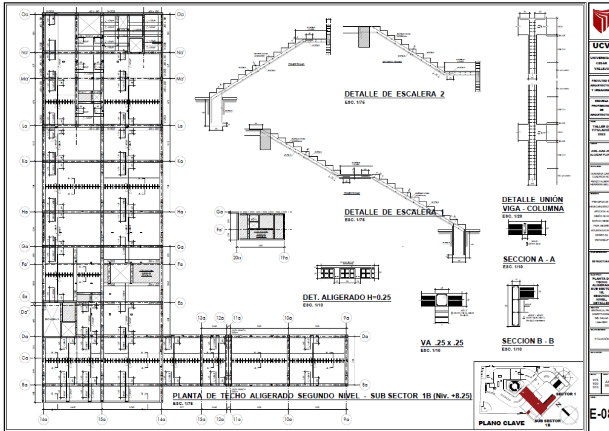
Planta de Techo Aligerado Segundo Nivel – Sub Sector 1B
