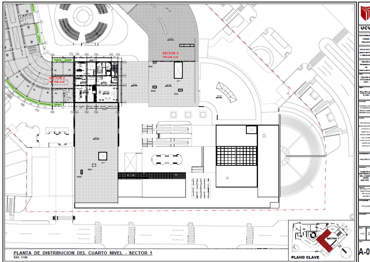
Planta de Distribución del Cuarto Nivel - Sector 1 (Esc. 1:125)
