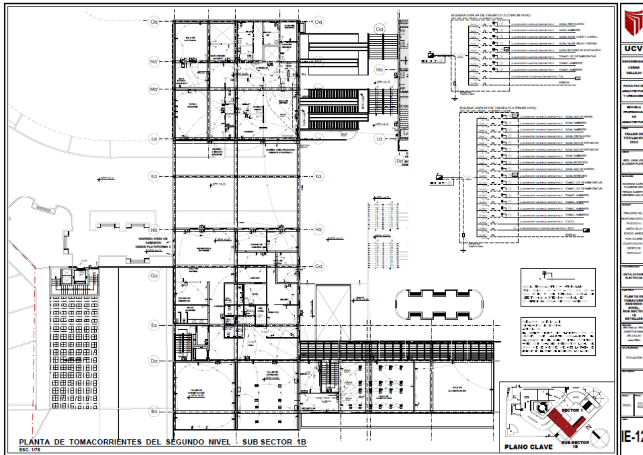
Planta de Tomacorrientes del Segundo Nivel – Sub Sector 1B
