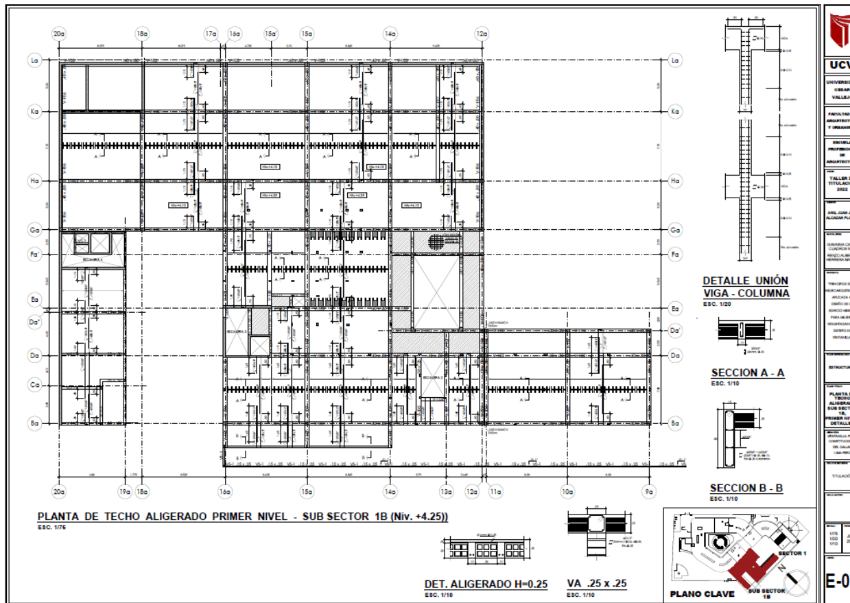
Planta de Techo Aligerado Primer Nivel – Sub Sector 1B
