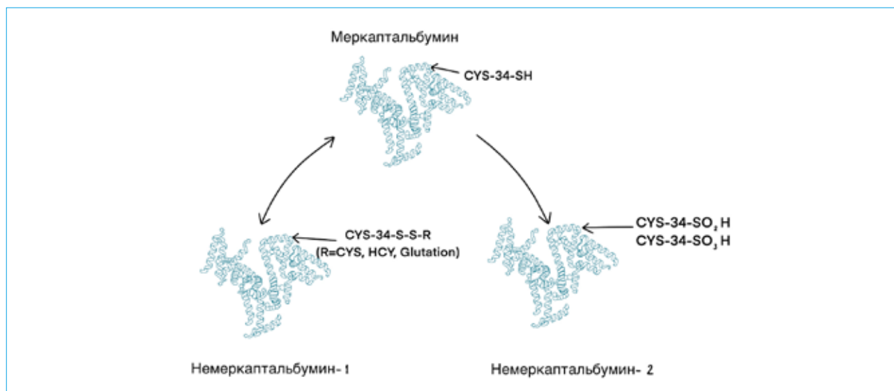
Рис. 2. Фракции альбумина. В зависимости от статуса Cys-34 альбумин может находиться в свободной, неокисленной форме — меркаптальбумин (на его долю приходится более 70 %), обратимо окисленной форме — немеркаптальбумин-1 и необратимо окисленной — немеркаптальбумин-2 (CYS — цистеин, HCY — гомоцистеин, \text{SO}_2\text{H} — сульфоновая кислота, \text{SO}_3\text{H} — сульфоновая кислота)
