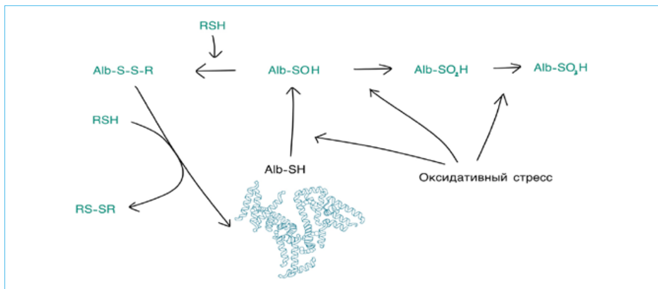
Рис. 4. Молекула сывороточного альбумина в условиях окислительного стресса. В физиологических условиях 2/3 молекул альбумина находятся в восстановленной форме со свободным остатком Cys-34 (Alb-SH) — меркаптальбумин. При окислительном стрессе Cys-34 окисляется с образованием сульфеновой кислоты (Alb-SOH). Сульфеновая кислота может быть окислена до конечных продуктов — сульфиновой (Alb-SO 2 H) или сульфоновой (Alb-SO 3 H) кислот либо превращена в дисульфид (Alb-SSR) с последующим возвращением в восстановленную форму — меркаптальбумин (Alb-SH)
