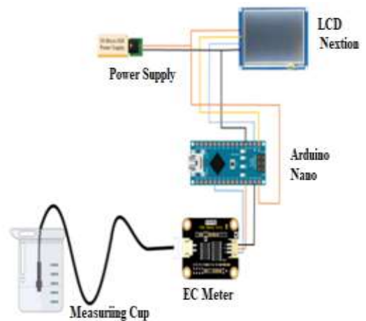
3a) Electrical wiring
