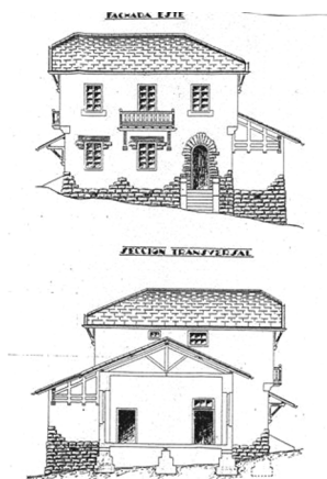
Martitteen eskolen proiektua
