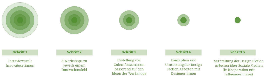
Abbildung 1: bio:fictions Prozess
