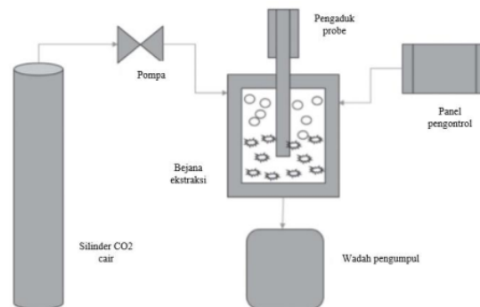
Gambar 5.14. Skema pabrik ekstraktor fluida superkritis. (Suleria and Barrow, 2020)
