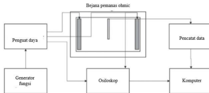
Gambar 5.11. Diagram skematik sistem ohmik frekuensi tinggi (Suleria and Barrow, 2020).
