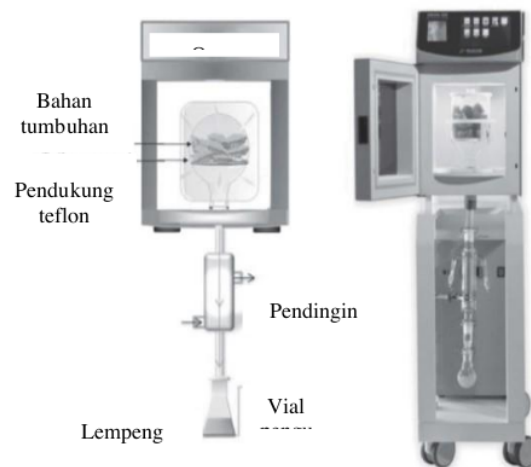
Gambar 5.10. Ekstraksi dengan sistem hidrodifusi microwave dan gravitasi (Suleria and Barrow, 2020)
