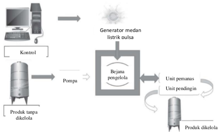
Gambar 5.13. Diagram skematis dari ekstraksi berbantuan medan listrik berdenyut.
