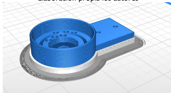
Figura 7 Vista archivo G-Code "generación de capas para imprimir el modelo 3D con una orientación de capa horizontal. Fuente: Elaboración propia los autores
