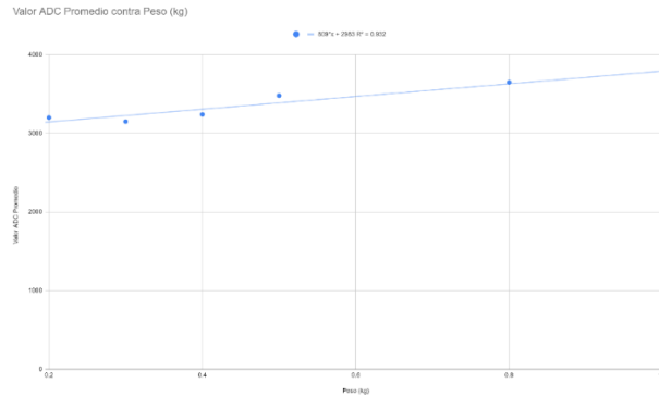
Figura 15 Comportamiento de los datos. Fuente: Elaboración propia
