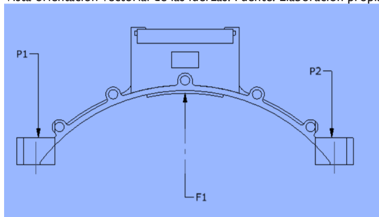
Figura 14 Montaje de pruebas en laboratorio. Fuente: Elaboración propia
