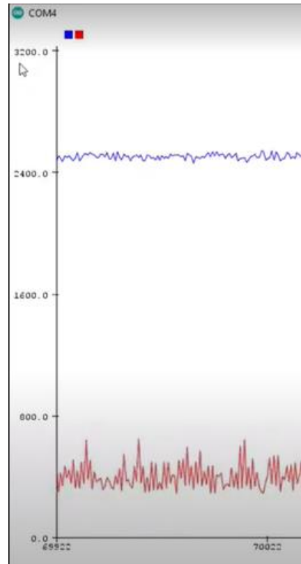
Figura 12 Arduino serial plotter comportamiento bits de entrada medias y varianza de datos. Fuente: Elaboración propia los autores
