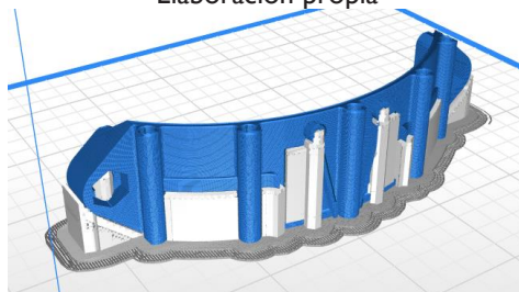
Figura 6 Vista archivo G-Code generación de capas para imprimir el modelo 3D con una orientación de capa vertical. Fuente: Elaboración propia
