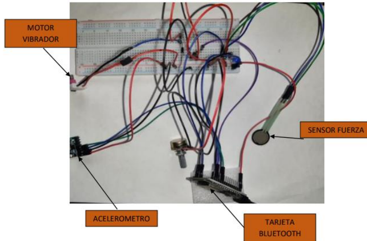
Figura 9 Montaje circuito eléctrico. Fuente: Elaboración propia los autores
