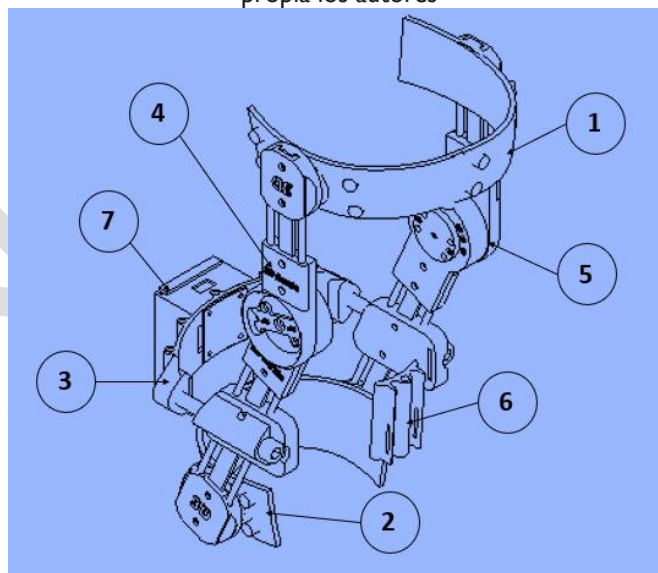
Figura 2 Vista isométrica versión I dispositivo externo para el tratamiento de ligamento cruzado posterior. Fuente: Elaboración propia los autores
