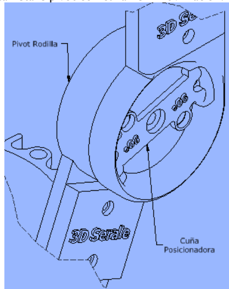
Figura 4 Vista isométrica detalle pivot con cuña de inmovilización. Fuente: Elaboración propia
