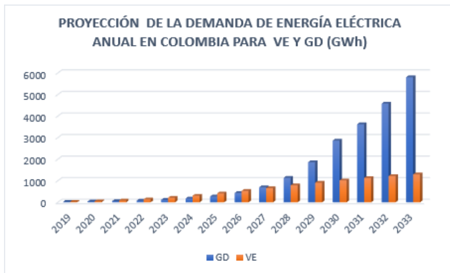
Figura 2. Proyección de la demanda de energía eléctrica anual en Colombia para vehículos eléctricos y generación distribuida
