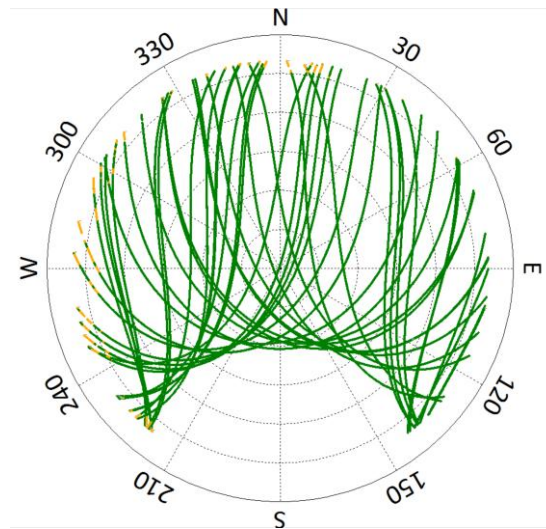
Figura 4. Skyplot. Máscara de elevación 7°. Figure 4. Skyplot. Elevation mask 7°.
