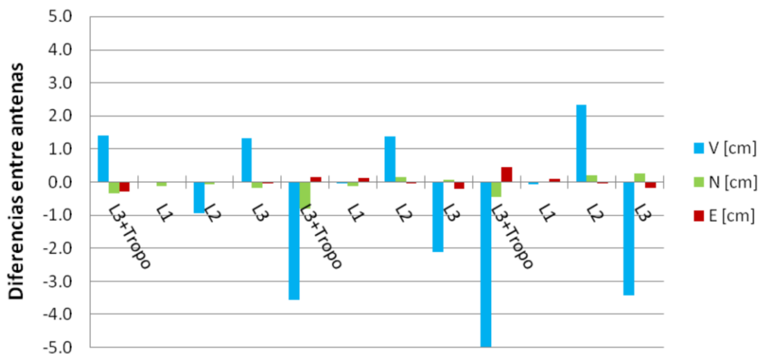
Figura 9. Comparación de posiciones entre las antenas con inclinación 0°. Figure 9. Comparison of positions between the antennas with tilt 0°.
