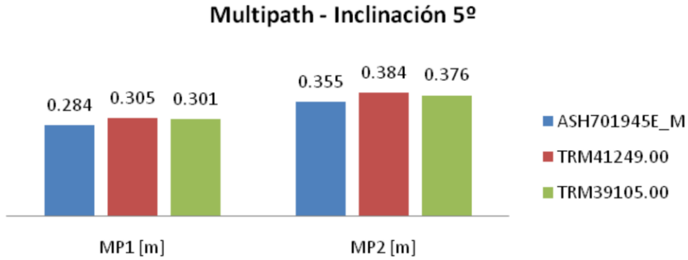
Figura 7. Multipath estimado para las 3 antenas con inclinación 5°. Figure 7. Estimated multipath of the 3 antennas with tilt 5°.
