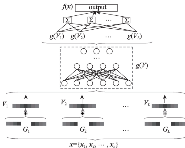
图 1 基本的 GSF 模型结构(以只含有三个文档的列表为例)
