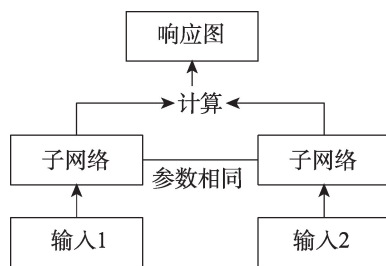
图2 孪生网络架构
