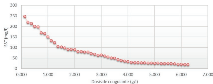
Figura 5 | Valores de SST obtenida posterior a los ensayos de prueba de jarra.
